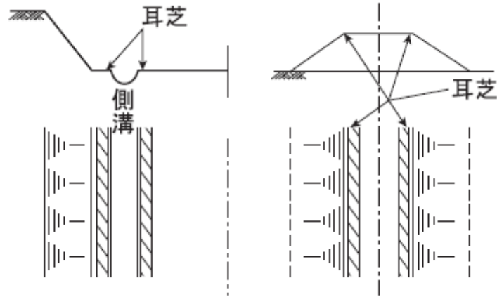
図2-6 耳芝
