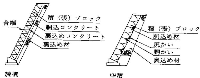
図2-5 コンクリートブロック工
