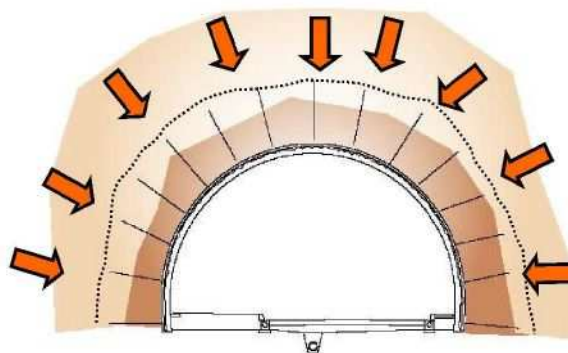
図3.2 NATMの工法概念図
