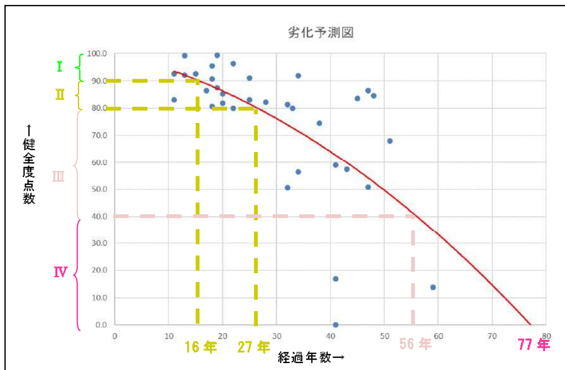
図7.1 劣化予測式
