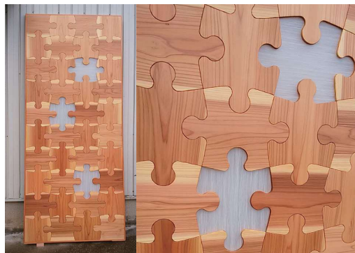
●木目を楽しむ工夫として製作したジグソーパズル形状の組木引戸
