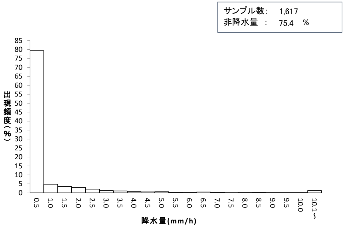
図Ⅲ－２－３ 時間降水量（0.5mm以上）度数分布（境港局、R06年度第1～3四半期まで）
