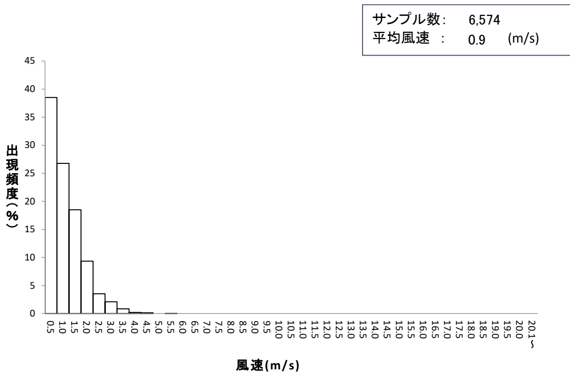
図Ⅲ－２－７ 風速度数分布（木地山局、R06 年度第 1～3 四半期まで）
