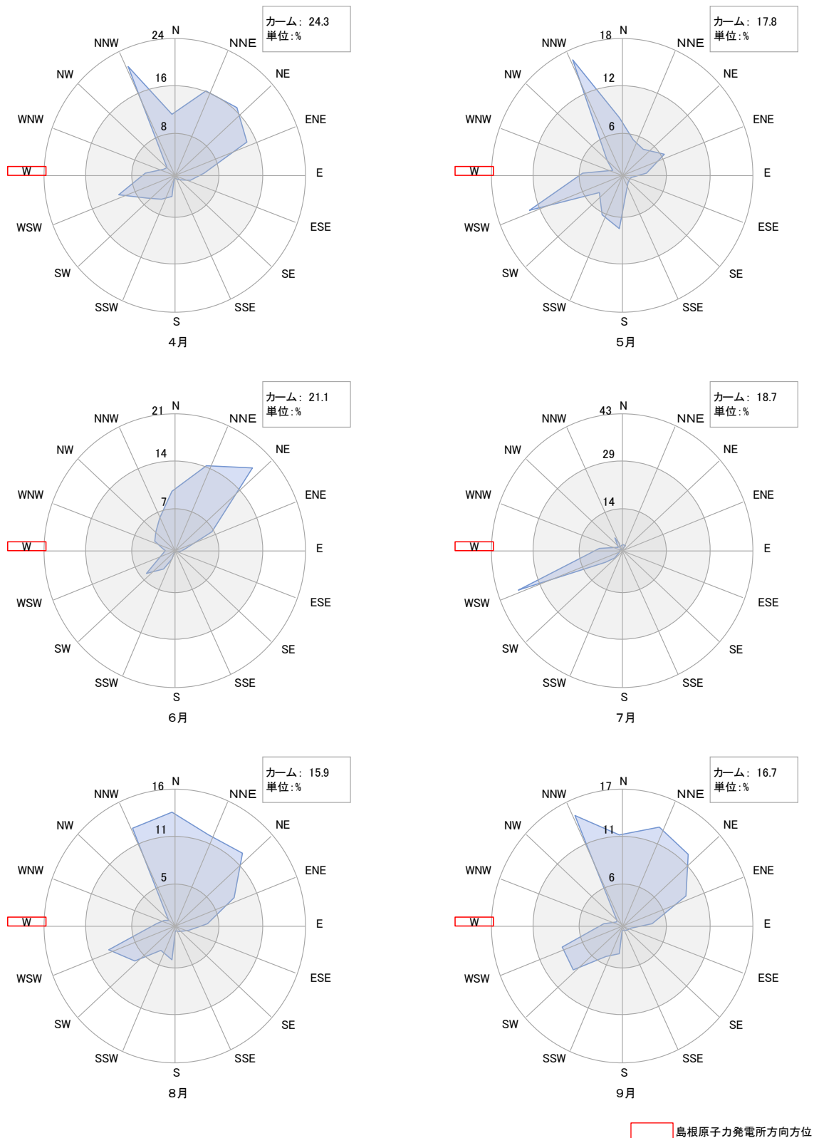
図Ⅲ-2-5-1 風配図（境港局、R06年度第1～2四半期まで）
