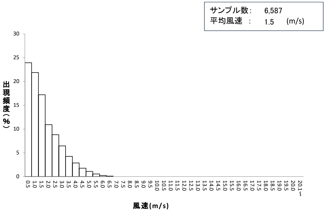
図Ⅲ－２－１ 風速度数分布（境港局、R06年度第1～3四半期まで）
