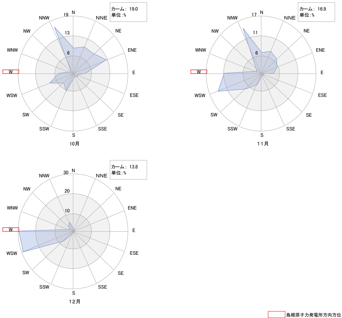
図Ⅲ－２－５－２ 風配図（境港局、R06年度第3四半期）
