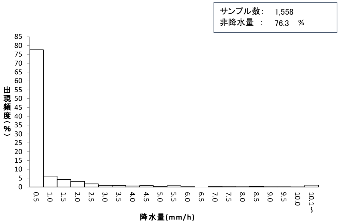
図Ⅲ－２－４ 時間降水量（0.5mm以上）度数分布（米子局、R06年度第1～3四半期まで）
