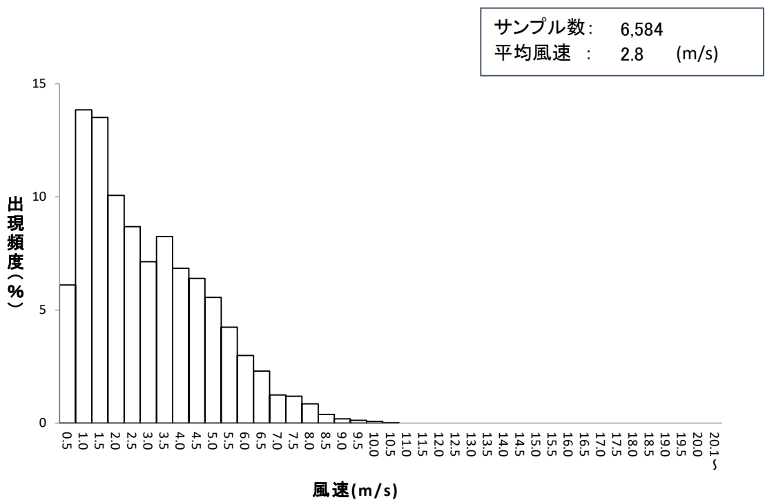
図Ⅲ－２－２ 風速度数分布（米子局、R06年度第1～3四半期まで）
