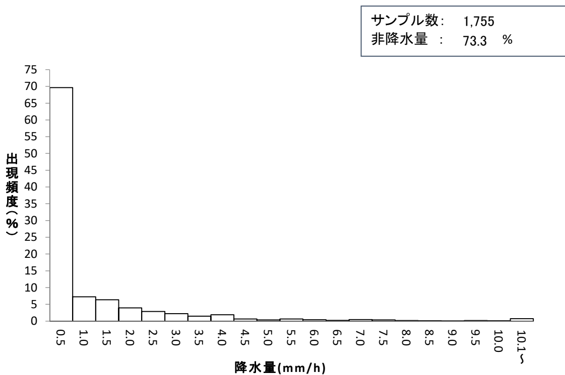
図Ⅲ－２－８ 降水量 (0.5mm/h 以上) 度数分布（木地山局、R06 年度第 1～3 四半期まで）
