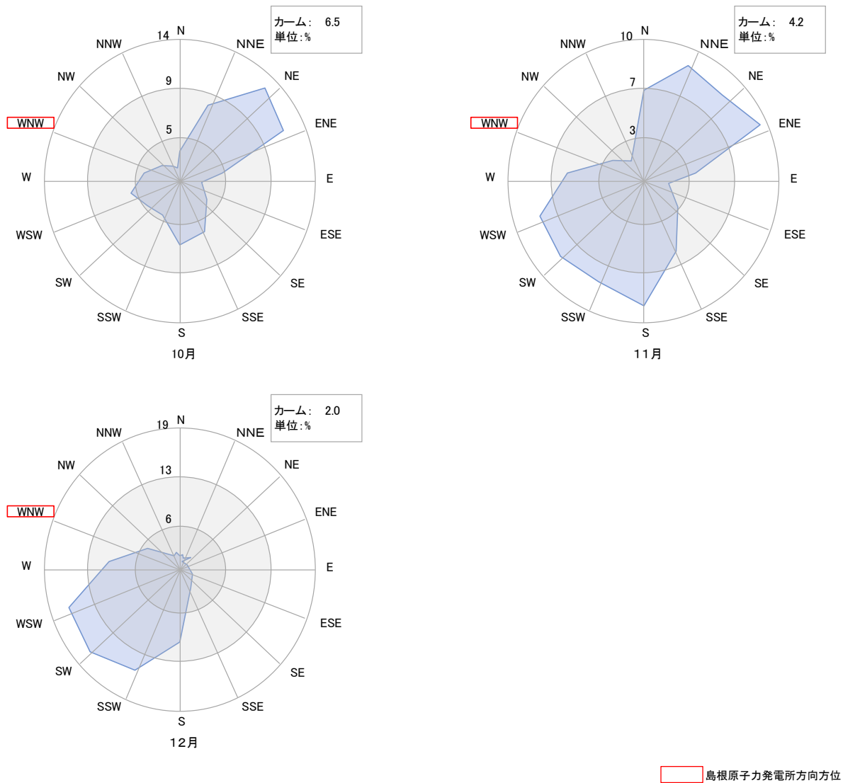
図Ⅲ-2-6-2 風配図 (米子局、R06 年度第3四半期)
