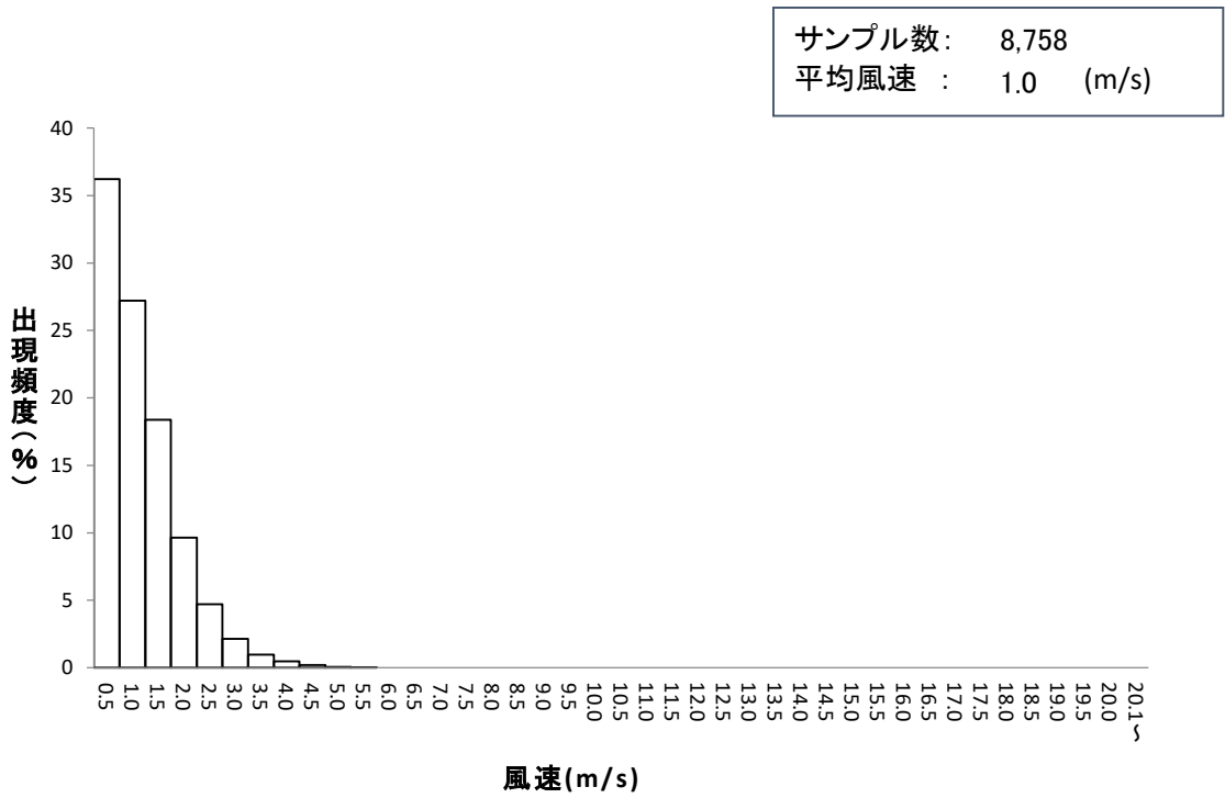
図IV-8-7 風速度数分布 (木地山局、R05 年度)
