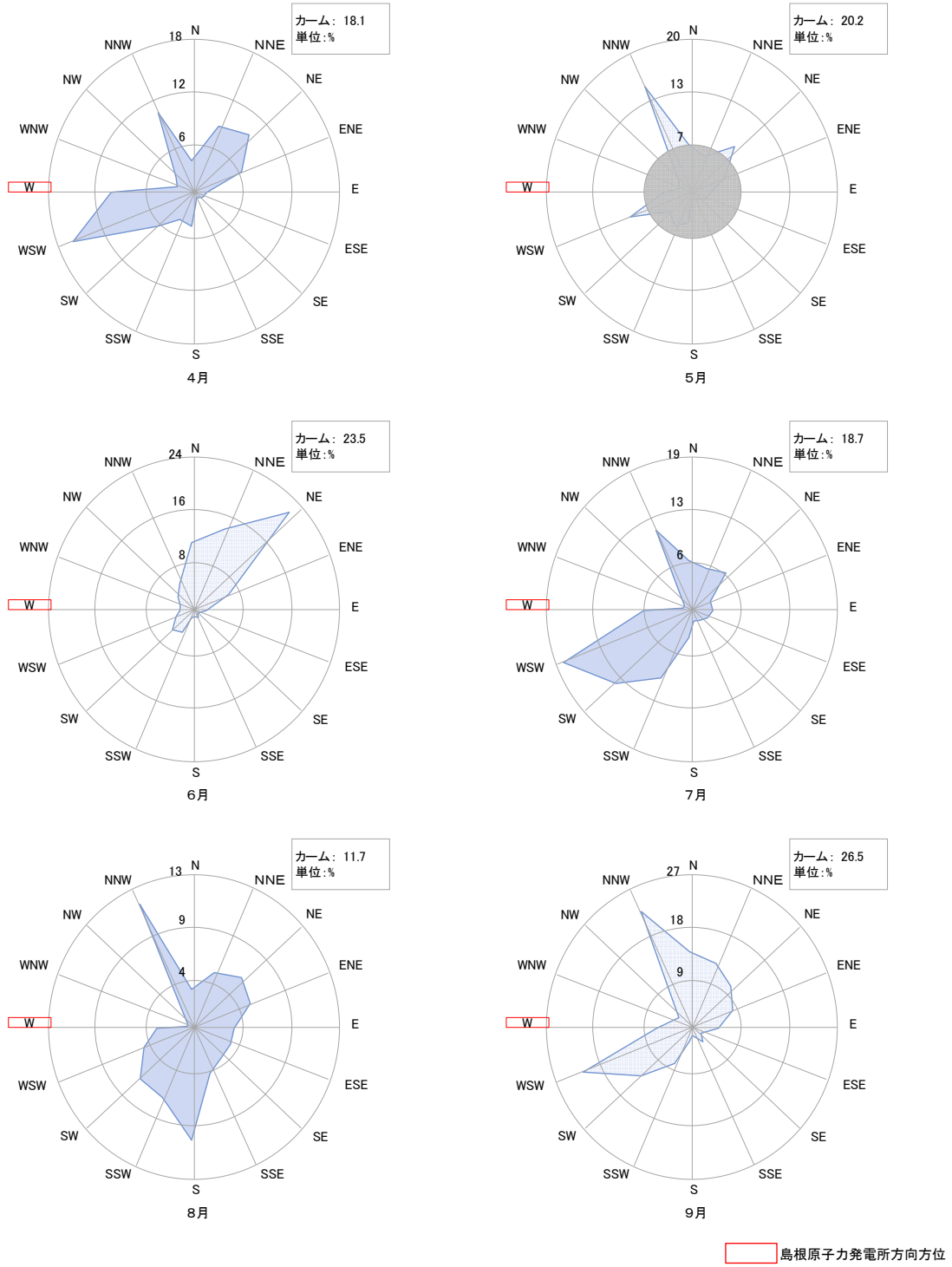
図IV-8-5-1 風配図 (境港局、R05年度)
