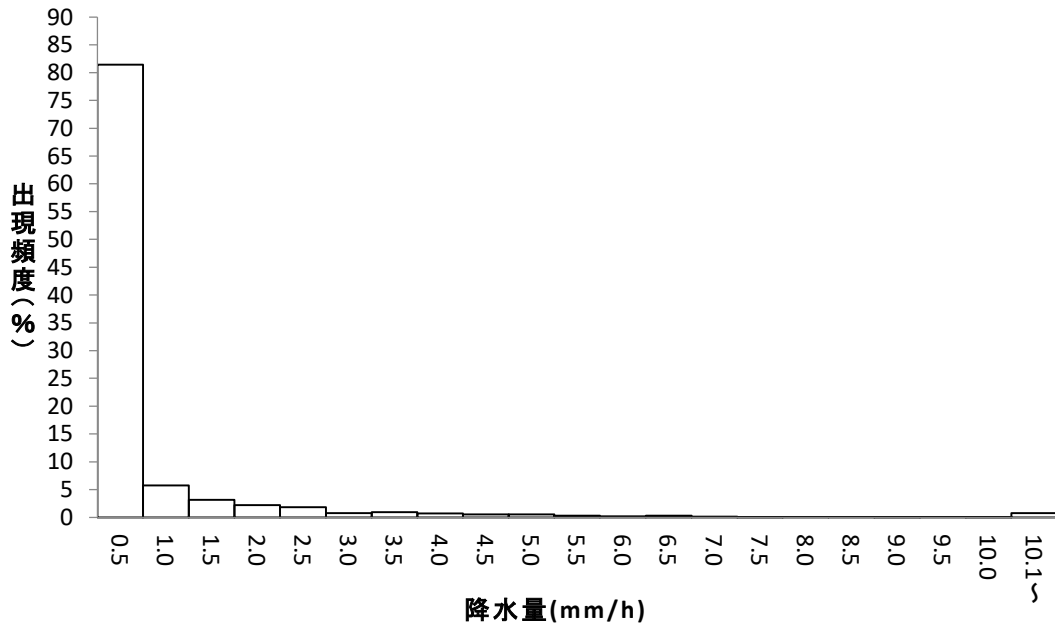
図IV-8-3 時間降水量(0.5mm以上)度数分布(境港局、R05年度)
