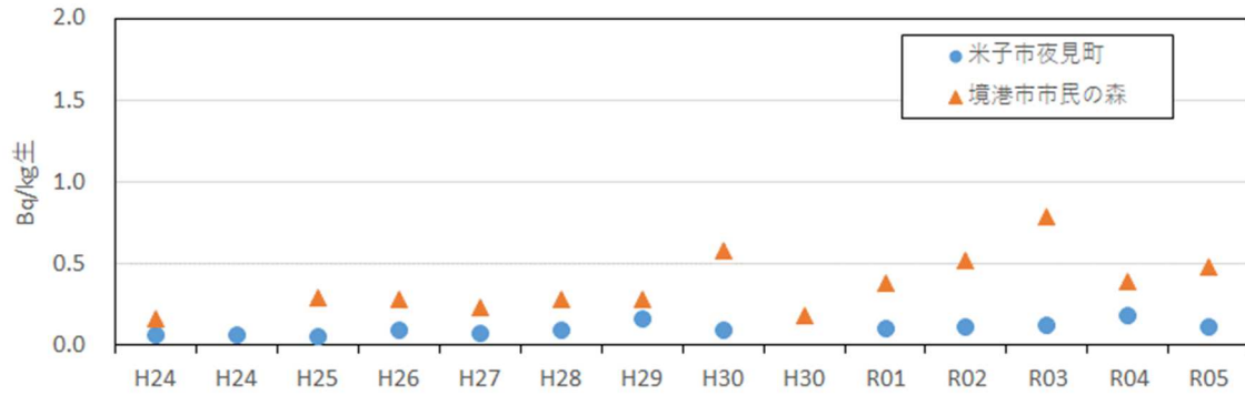
図IV-3-4 松葉中のセシウム 137 濃度の経時変化 (H24 年度から調査開始)
