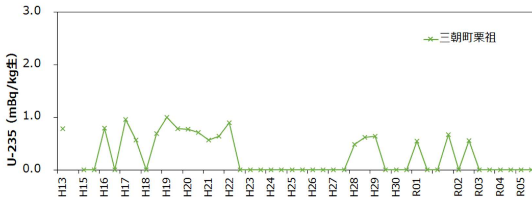
図IV-5-3 植物（杉葉）中のウラン235濃度の経時変化
