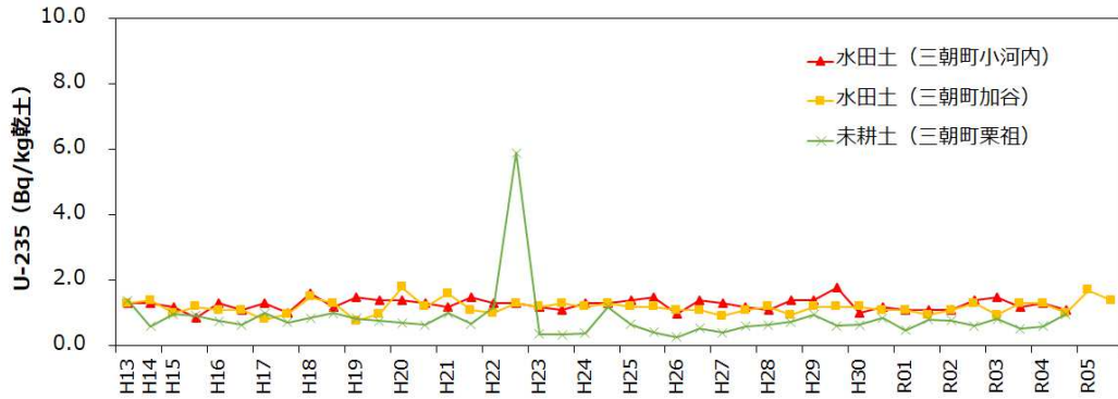
図IV-5-1 土壌（水田土、未耕土）中のウラン235濃度の経時変化
