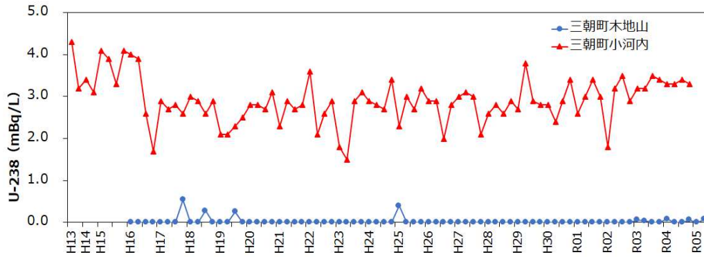
図IV-5-4 陸水中のウラン 238 濃度の経時変化
