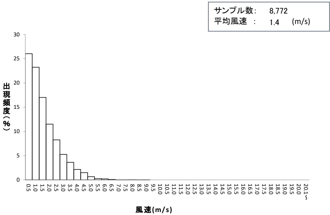
図IV-8-1 風速度数分布 (境港局、R05 年度)
