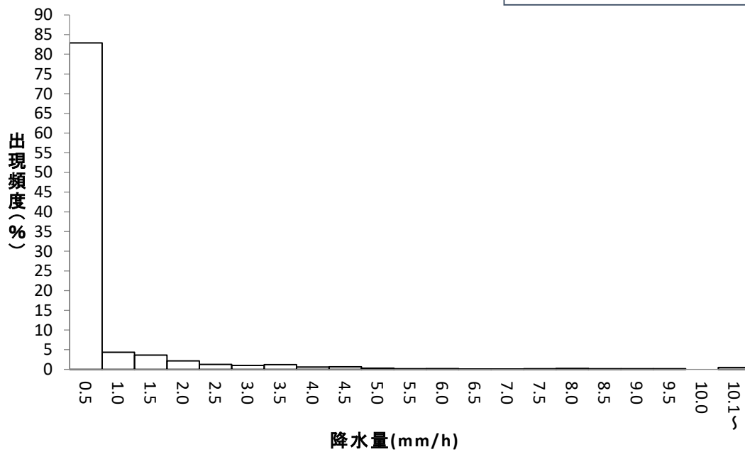
図IV-8-4 時間降水量(0.5mm以上)度数分布(米子局、R05年度)
