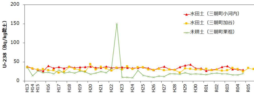
図IV-5-5 土壌 (水田土、未耕地) 中のウラン 238 濃度の経時変化
