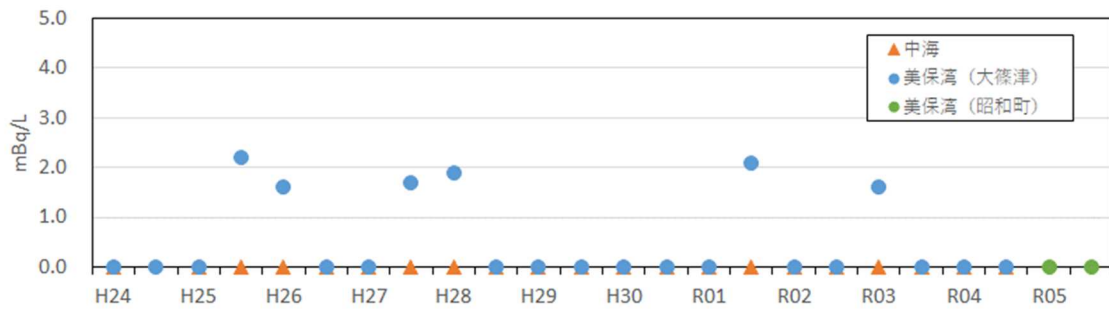
図IV-3-6 海水中のセシウム 137 濃度の経時変化 (H24 年度から調査開始)
