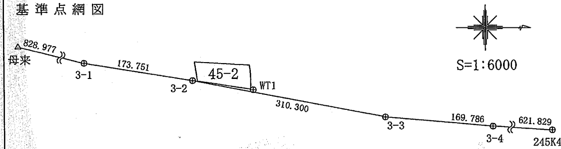
3級基準点：ネットワーク型RTK法による基準点測量
