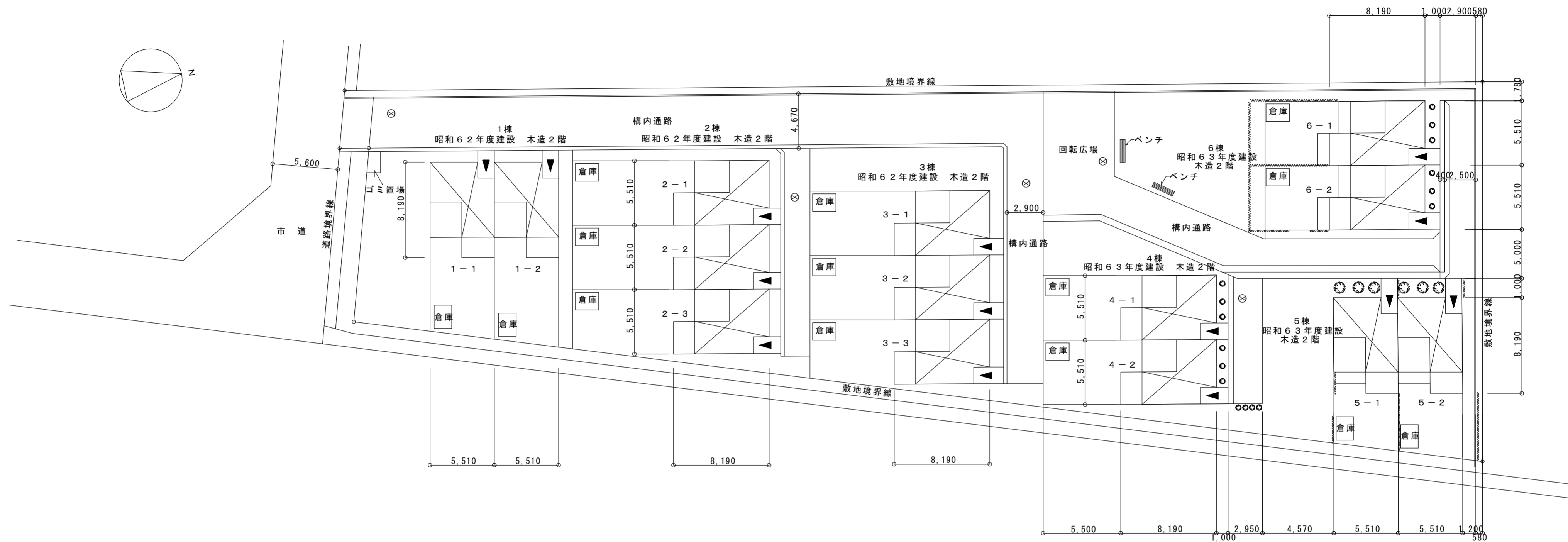
配置図 S=1:250
