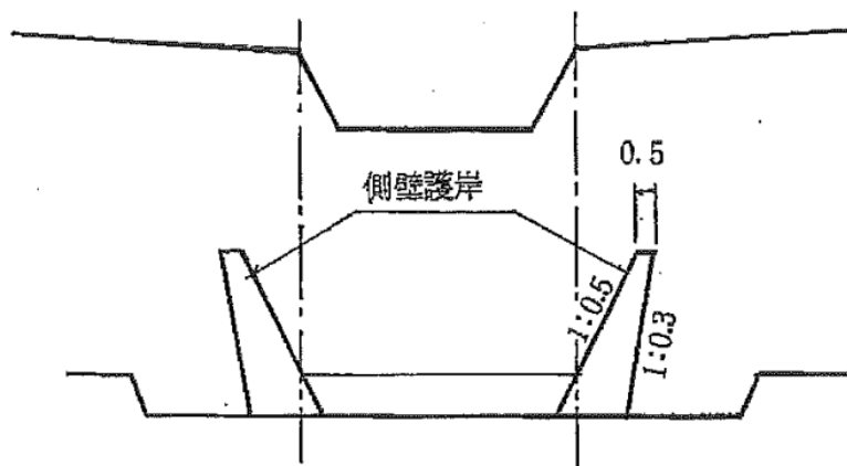
図4-2-1 主えん堤部側壁位置図
