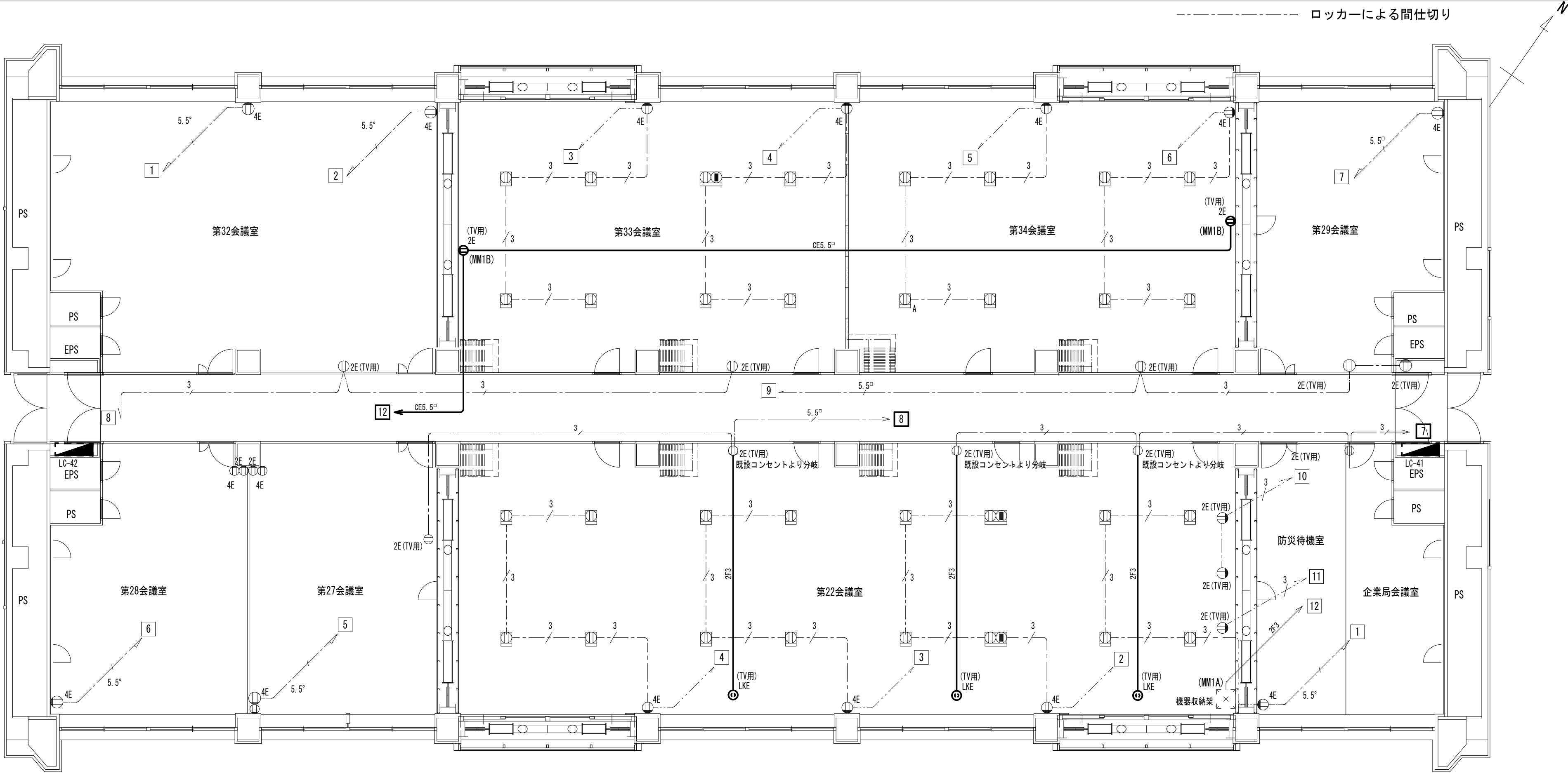
【更新後】コンセント設備 4階 配線図 S=1/100
