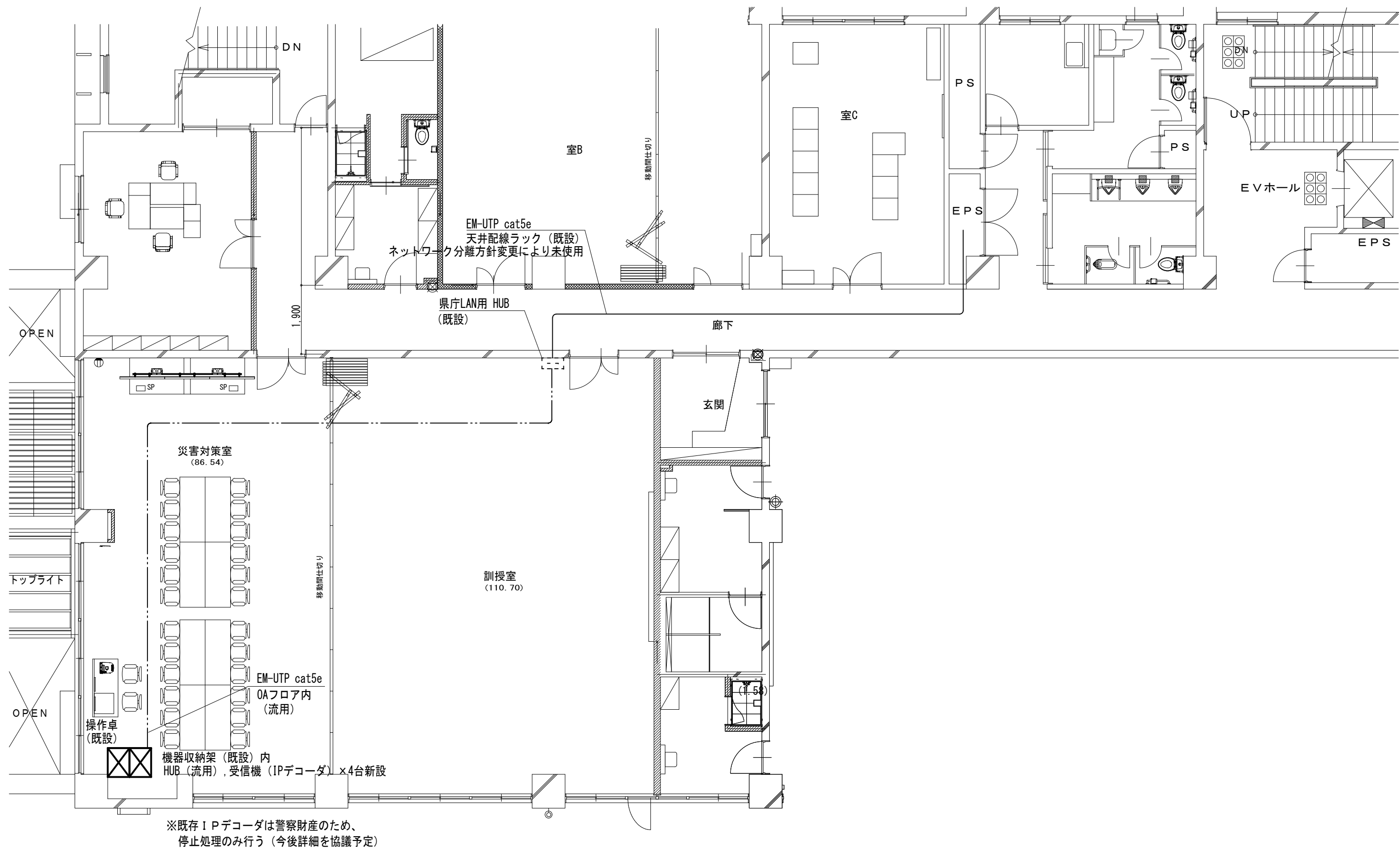
映像音響設備 3階 更新図、撤去図 S=1/100
