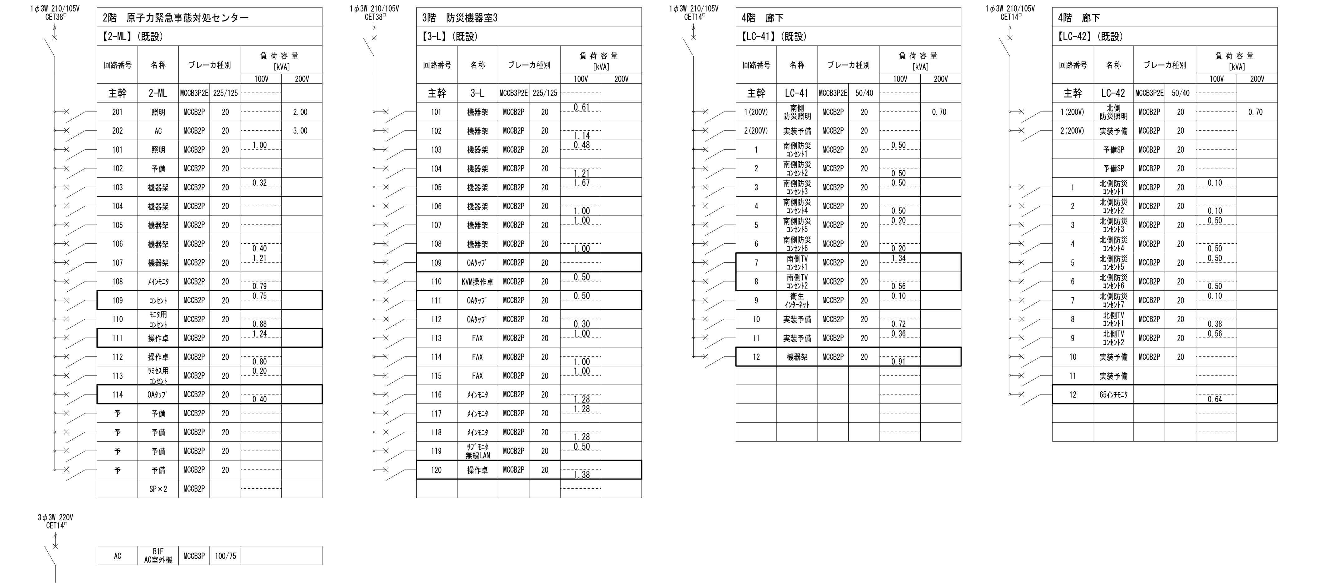
電灯分電盤結線図（分電盤改修なし、既設ブレーカへ新設配線接続）
