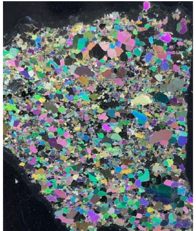
写真3 偏光顕微鏡で見たかんらん岩（秋田県一ノ目瀧産）。写真の横幅はおよそ20mm。
