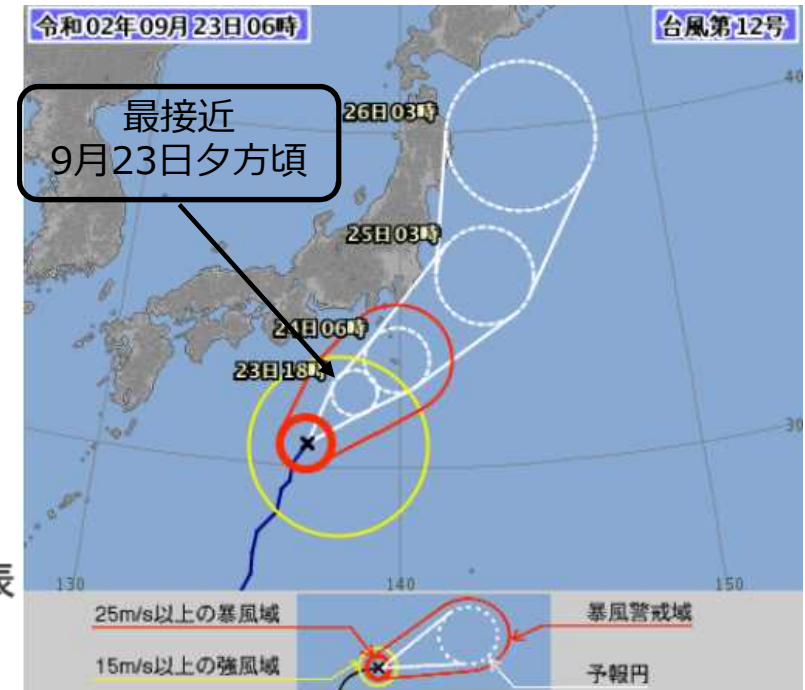
台風進路予想（23日06時）
