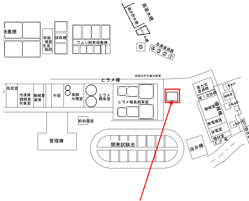
井戸海水ポンプ4-1号機位置
