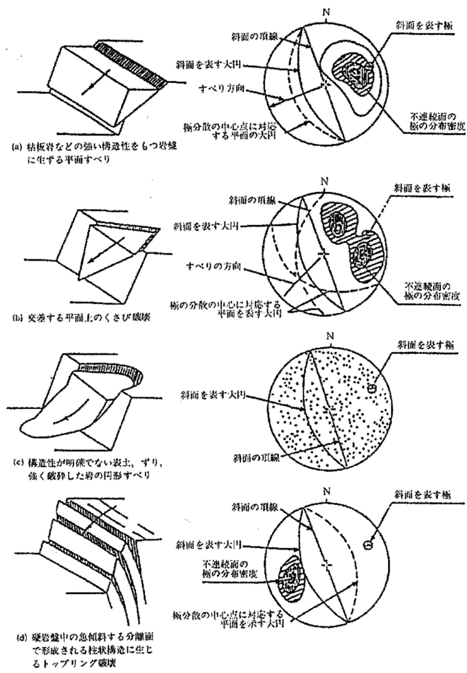
図 2-4 割れ目分布パターンと斜面崩壊タイプ
