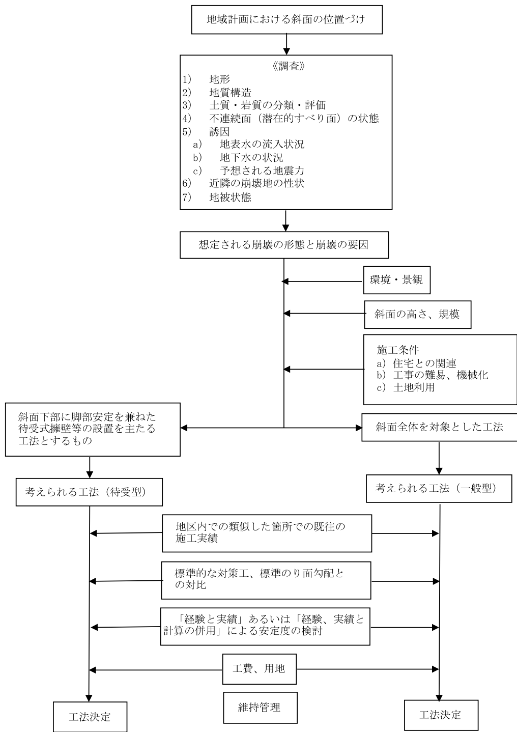
図 2-5 工法選定のフローチャート
