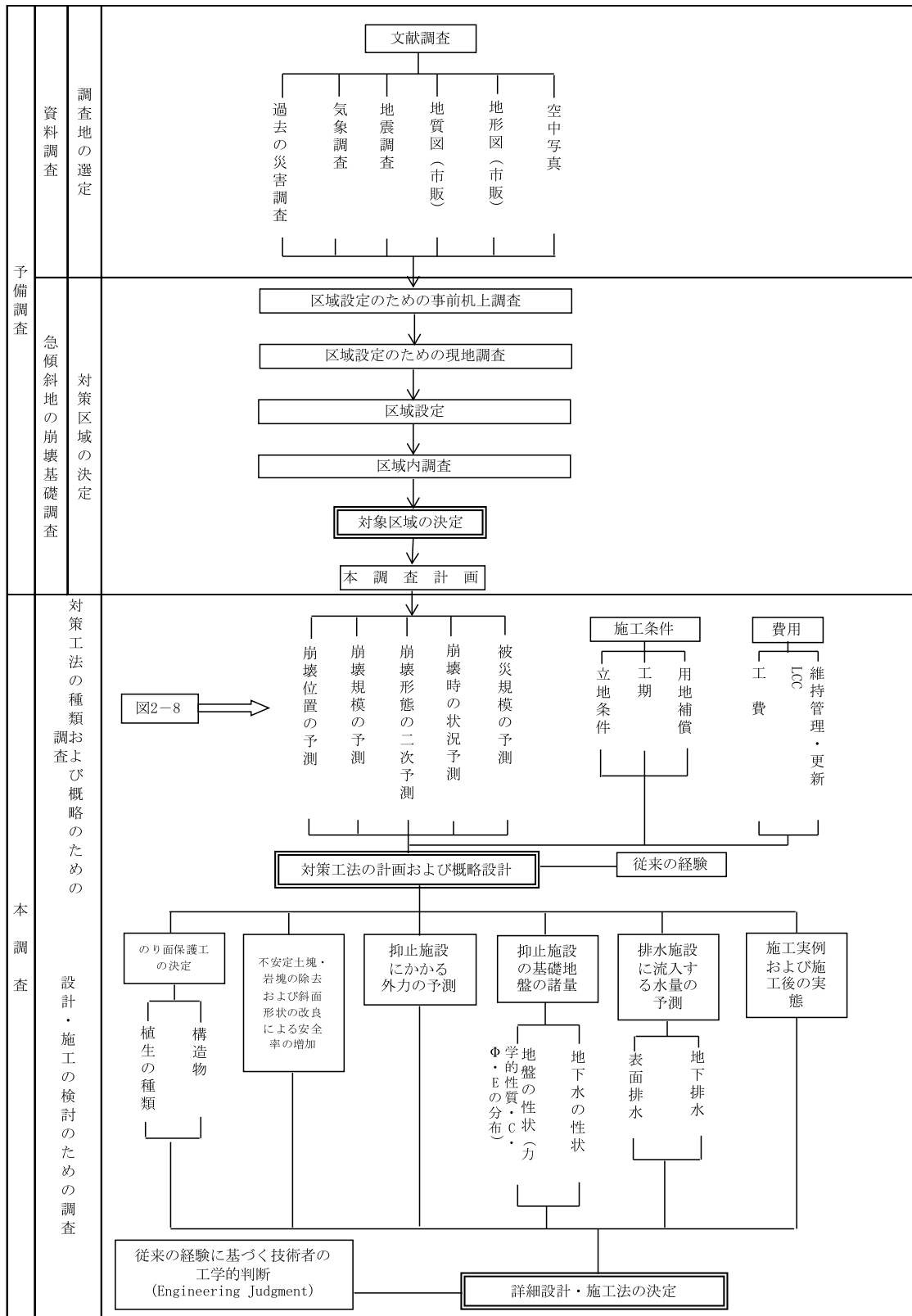
図 2-1 斜面調査の種類と流れ
