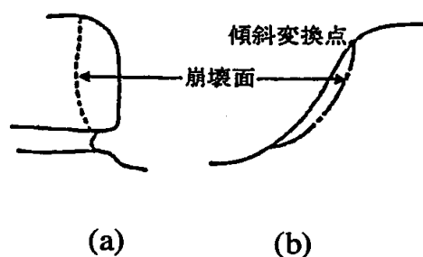
図 2-3 崩壊面の想定
