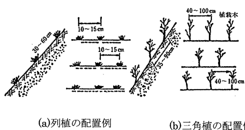
図 5-4 植栽配列の例
