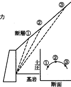
図 8-10 試行くさび法による土圧の算定
