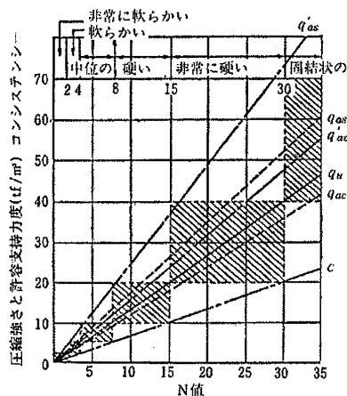
図 8-2 N 値と粘土のかたさ、一軸圧縮強さおよび許容支持力度との関係 (テルツァギ・ペック)
