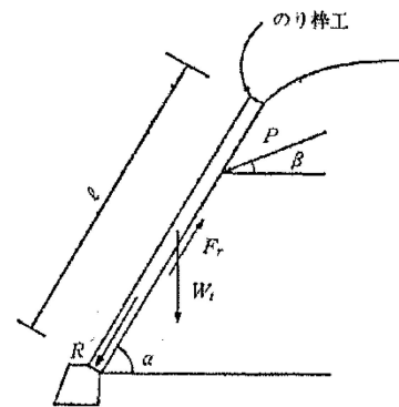
図8-42 のり枠工の基礎擁壁工
