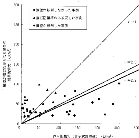
図 8-33 擁壁被災事例における作用衝撃力と計算上の限界耐力
