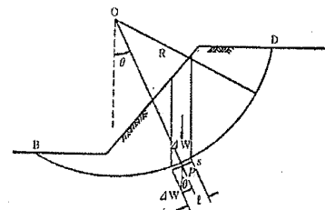
図 8-8 円弧すべりの安全解析
