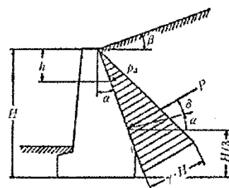
図 8-12 クーロン公式による 土圧算定のモデル
