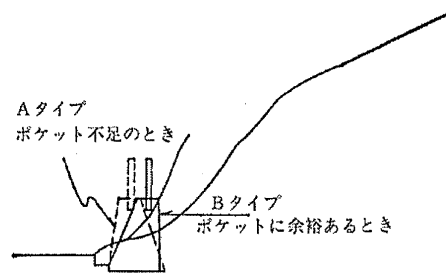
図 8-31 待受式コンクリート擁壁の裏勾配
