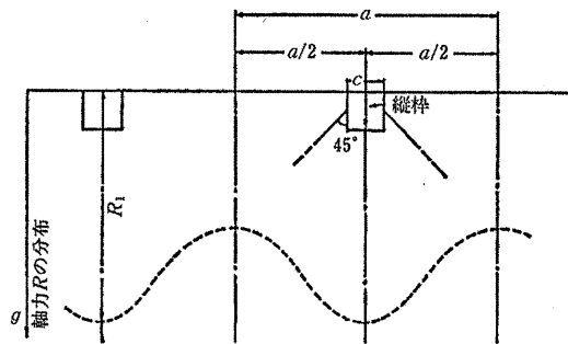
図 8-43 軸力(R)の分布
