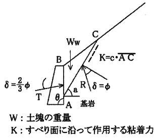
b. 粘着力を考慮した場合のくさびの考え方
