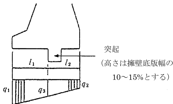
図 8-16 地盤反力度および水平距離のとり方
