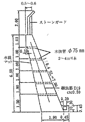
図 8-28 もたれコンクリート擁壁工の一例
