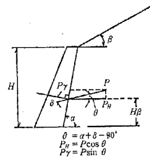
図 8-29 もたれコンクリート擁壁に作用する土圧
