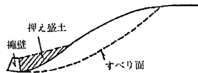
図 8-27 押え盛土の擁壁
