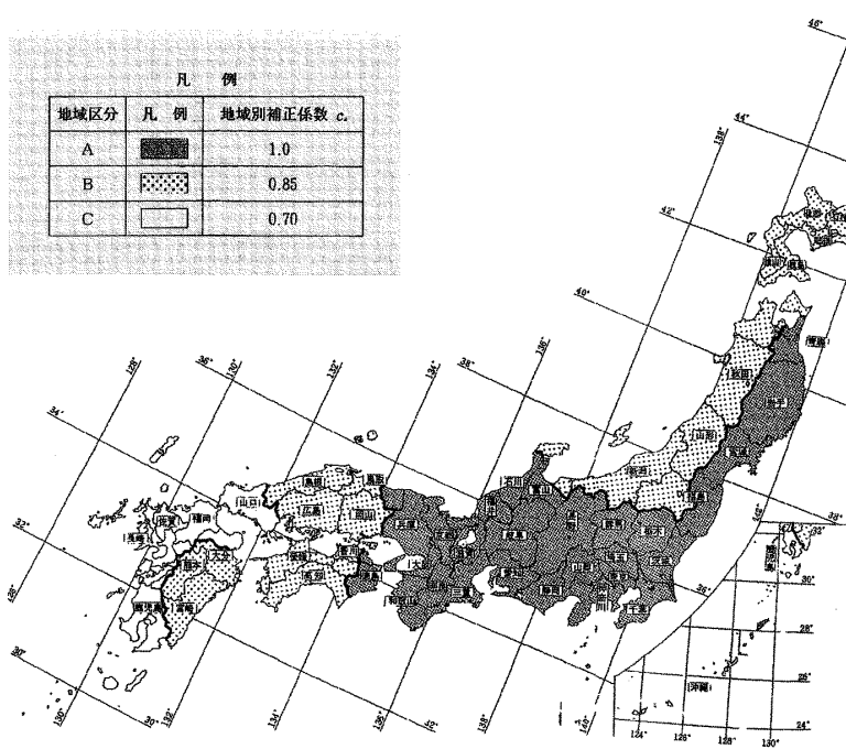
図 8-14 地域別補正係数
