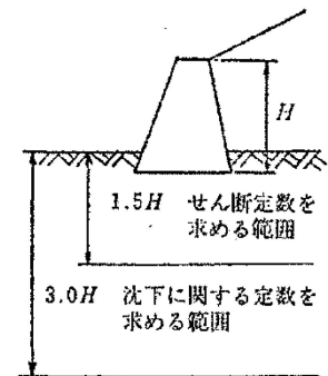
図8-1 調査すべき深さ
