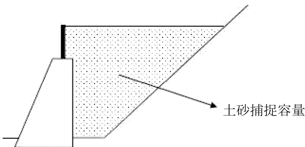
図8-37 単位幅当たりの土砂捕捉容量
