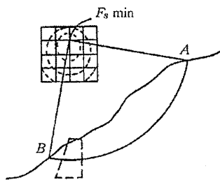
図 8-7 最小安全率を与えるすべり面
