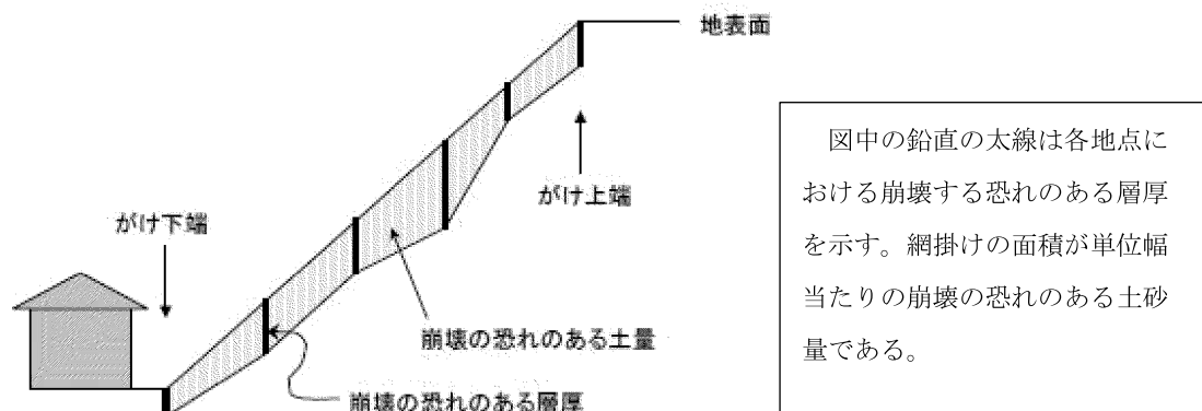
図8-35 崩壊土砂量算出の算定図
