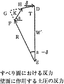
図 8-9 直線すべり土塊からの土圧の解析
