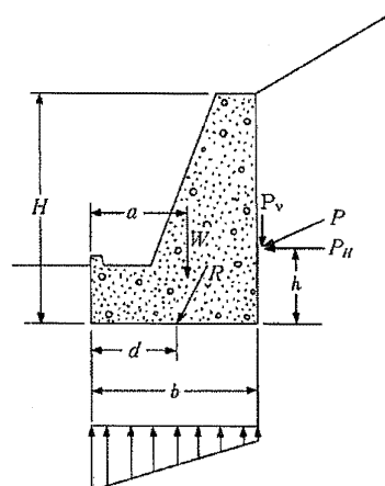
図 8-24 擁壁に作用する力
