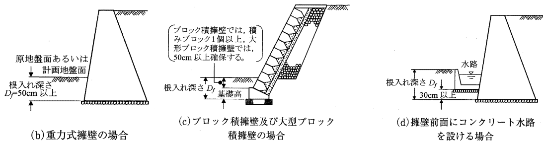
図8-41 擁壁工の直接基礎の根入れ深さ (出典：擁壁工指針p.129)
