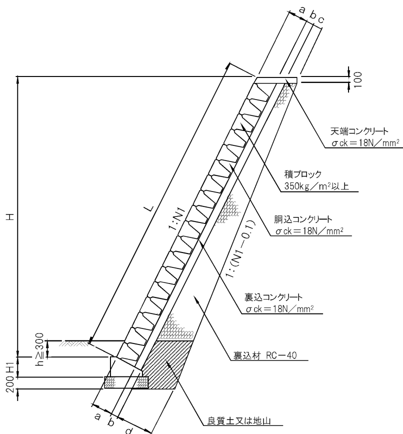
図 8-19 ブロック積擁壁の標準断面 (出典：小構造物標準設計図集 (鳥取県県土整備部))
