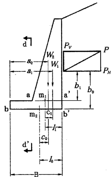
図 8-26 設計計算のための擁壁のモデル
