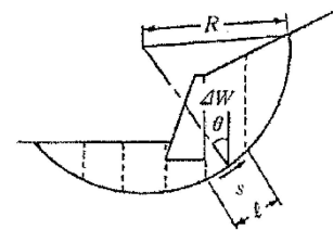
図 8-25 擁壁を含む全体の安定
