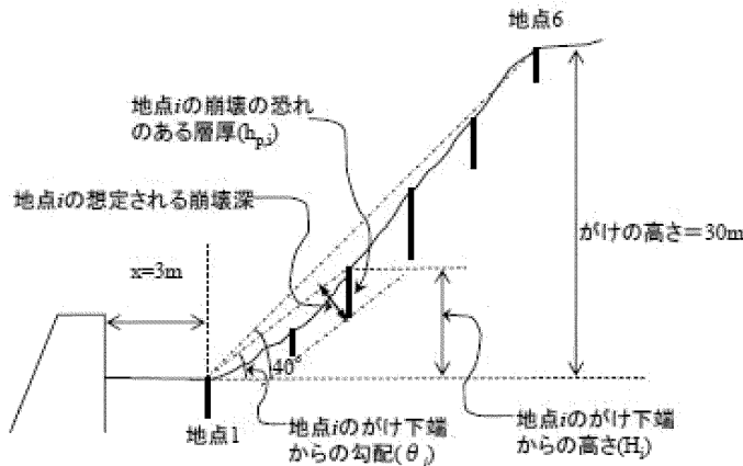
図8-36 検討斜面の模式図
