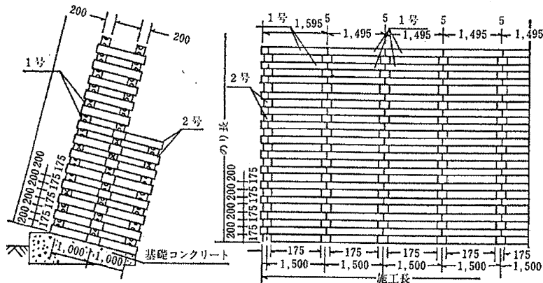
図 8-40 井桁組擁壁工の一例 (単位 : mm)
