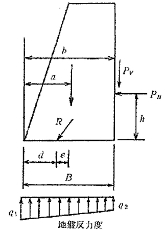
図 8-17 地盤反力度の求め方
