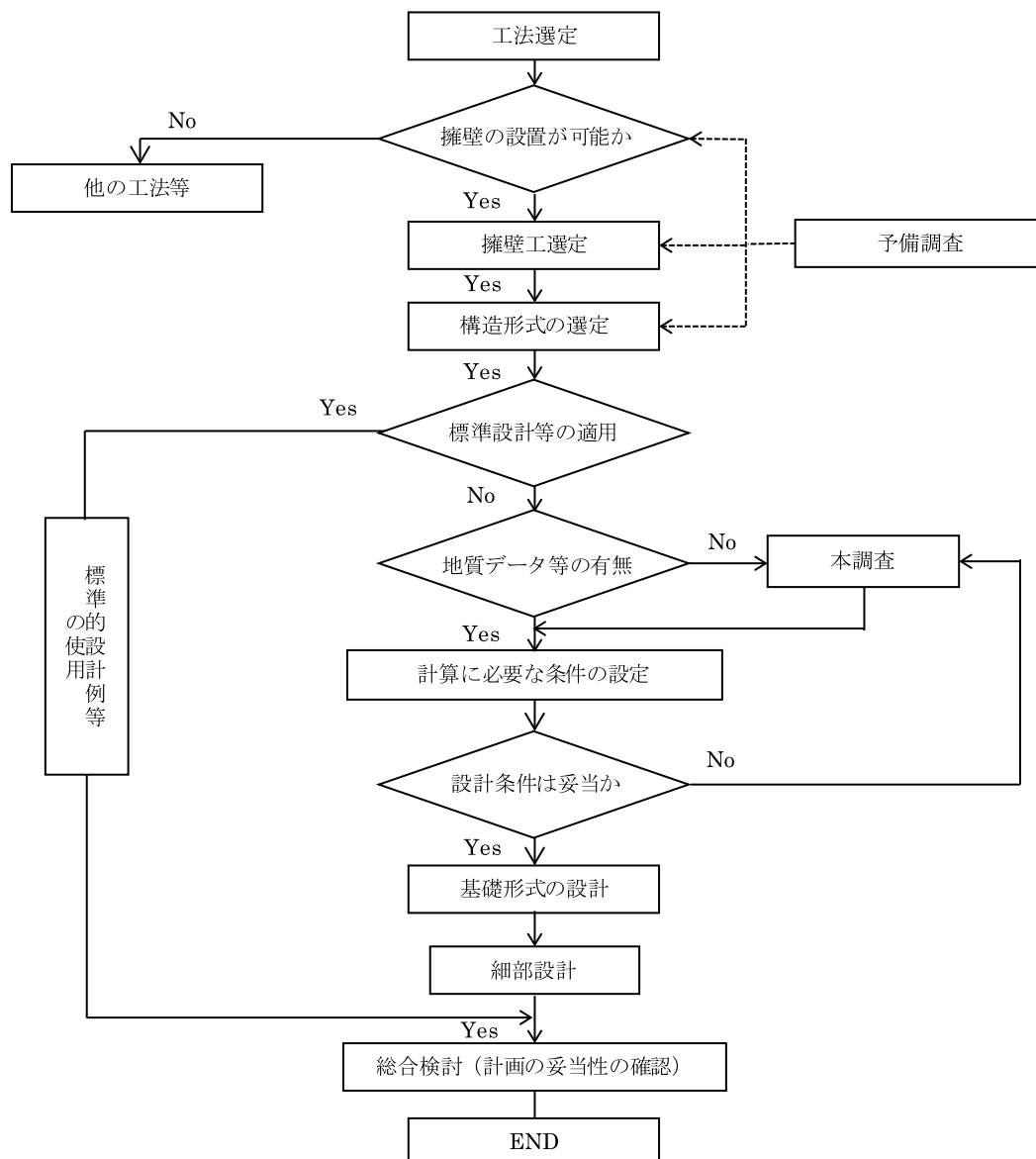
図 8-4 擁壁工の設計の手順の一例
