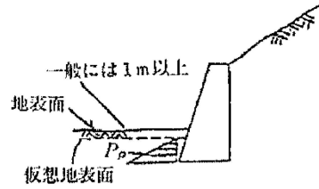
図 8-15 擁壁全面の受働土圧
