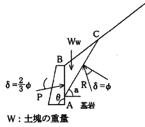
b. 粘着力を考慮した場合のくさびの考え方
