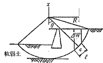
図8-3 すべり面
