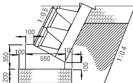
図 8-20 基礎工の設計標準の一例（出典：小構造物標準設計図集（鳥取県県土整備部））
