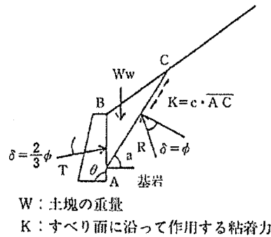
図 8-9 直線すべり土塊からの土圧の解析
