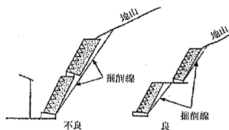
図8-21 多段式石積擁壁
