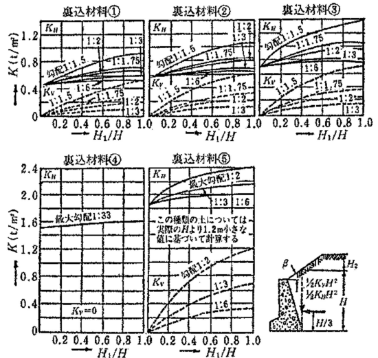
図 8-11 盛土部擁壁の設計に用いる土圧図
