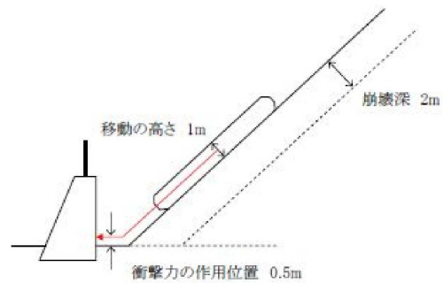
図 8-34 衝撃力の作用模式図
