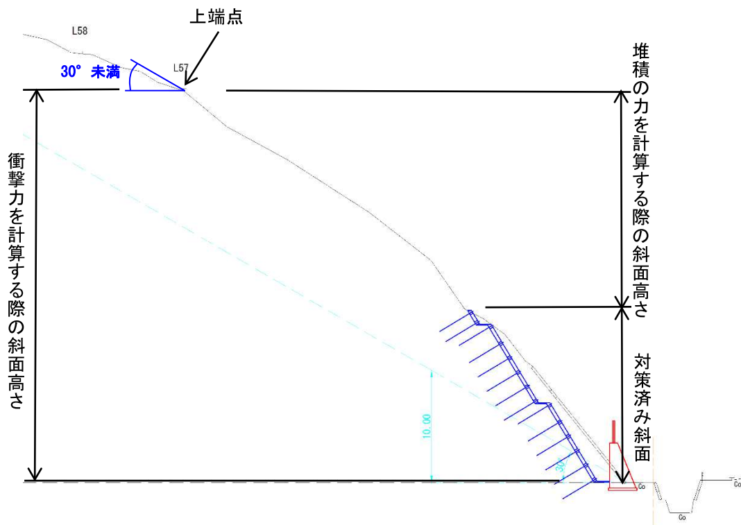
図8-32 設計計算時の斜面高さ
