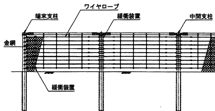
図 8-38 支柱強化型の防護柵
