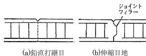
図 8-18 鉛直打継目および伸縮目地
