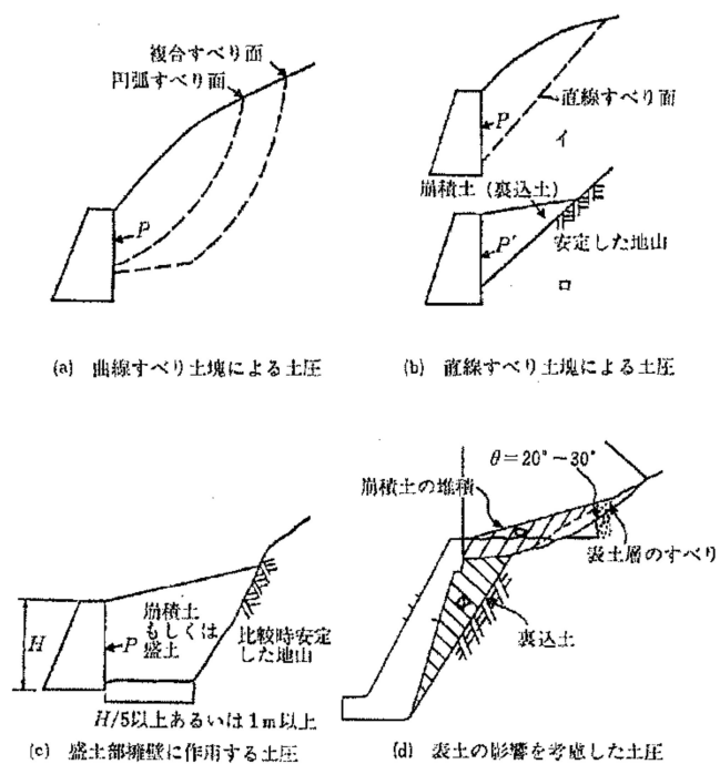
図 8-5 斜面における土圧の分類
