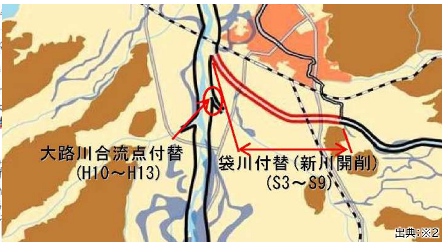
大路川流域の治水事業
