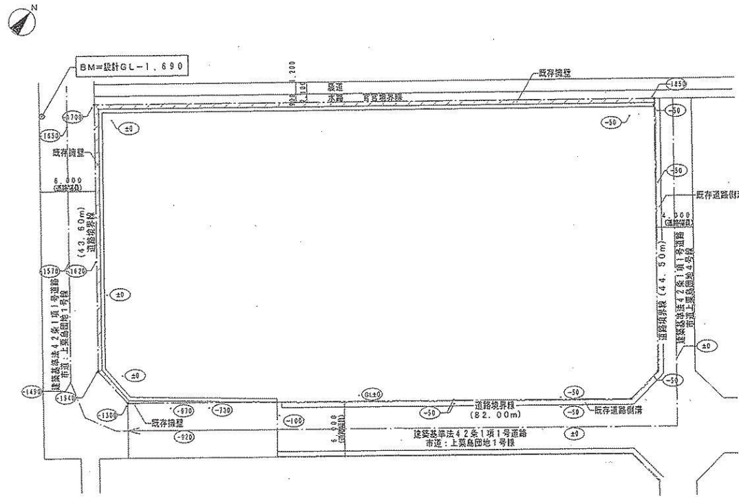
配置図 (1/400)
