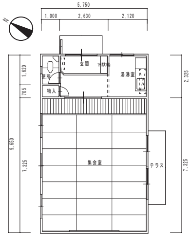
集会所(2)平面図 S=1:100
