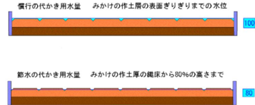
代かき用水量の設定の概要図（断面）
