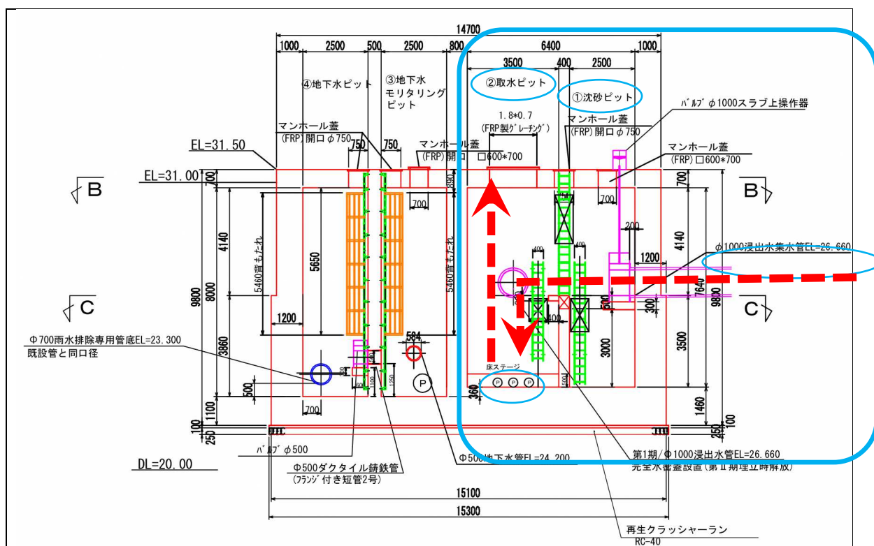
B：集水ピットの構造図
