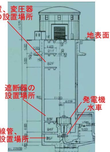
<発電所断面図>
