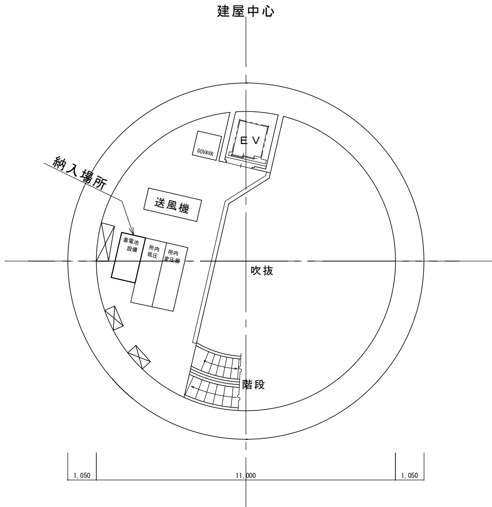
B 2 F 平面図 ( 1 / 1 0 0 )
