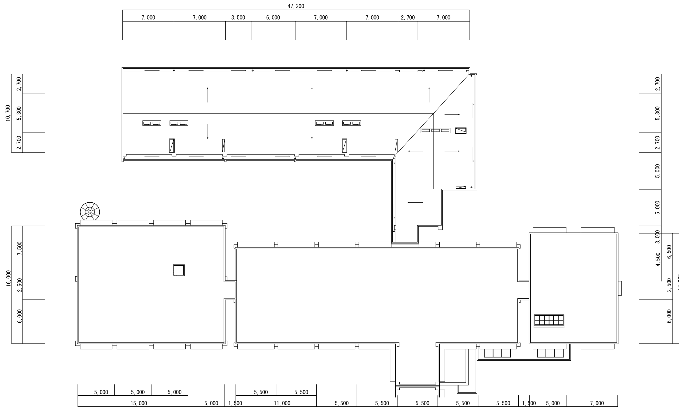
R階平面図 S=1/300
