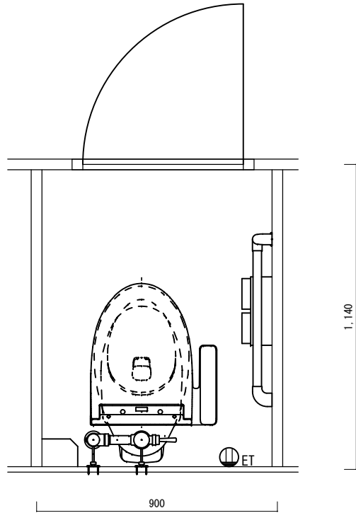
第二庁舎基準階トイレ詳細図（改修後） S=1:20
