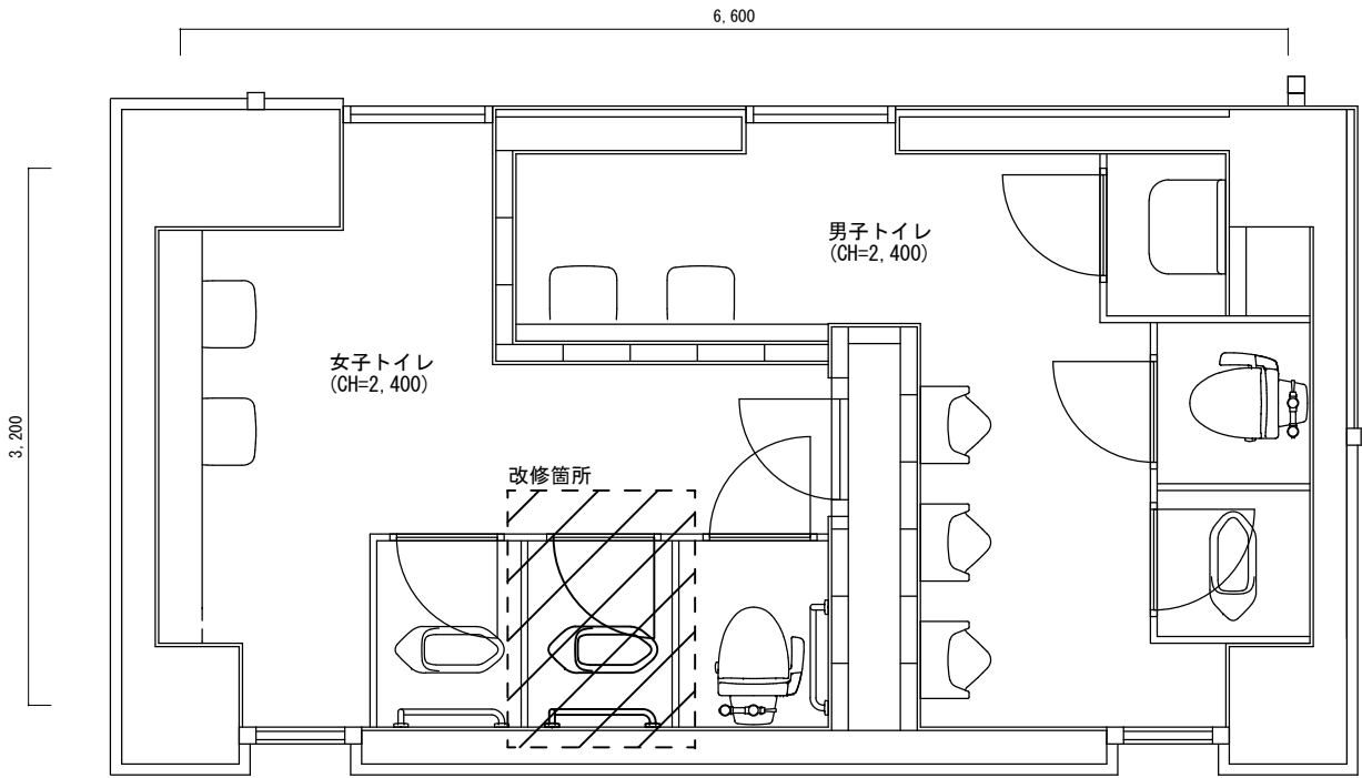
第二庁舎基準階トイレ平面図 S=1:50
