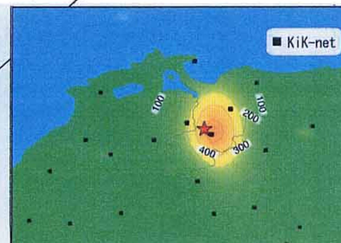
図3-3 観測地震動 (k-net および kik-net)
