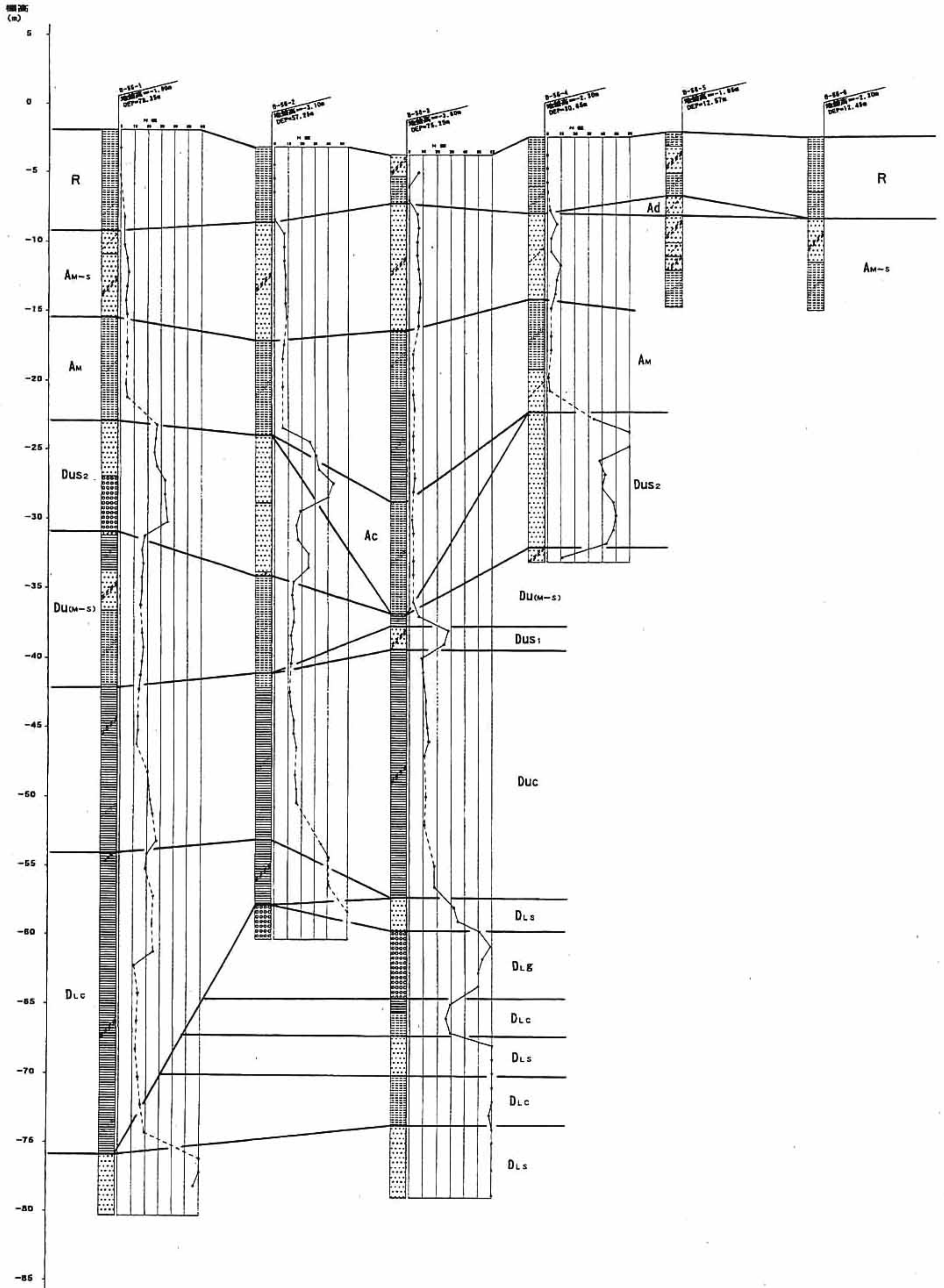
竹内工業団地柱状図一覽圖(S.56-1)
