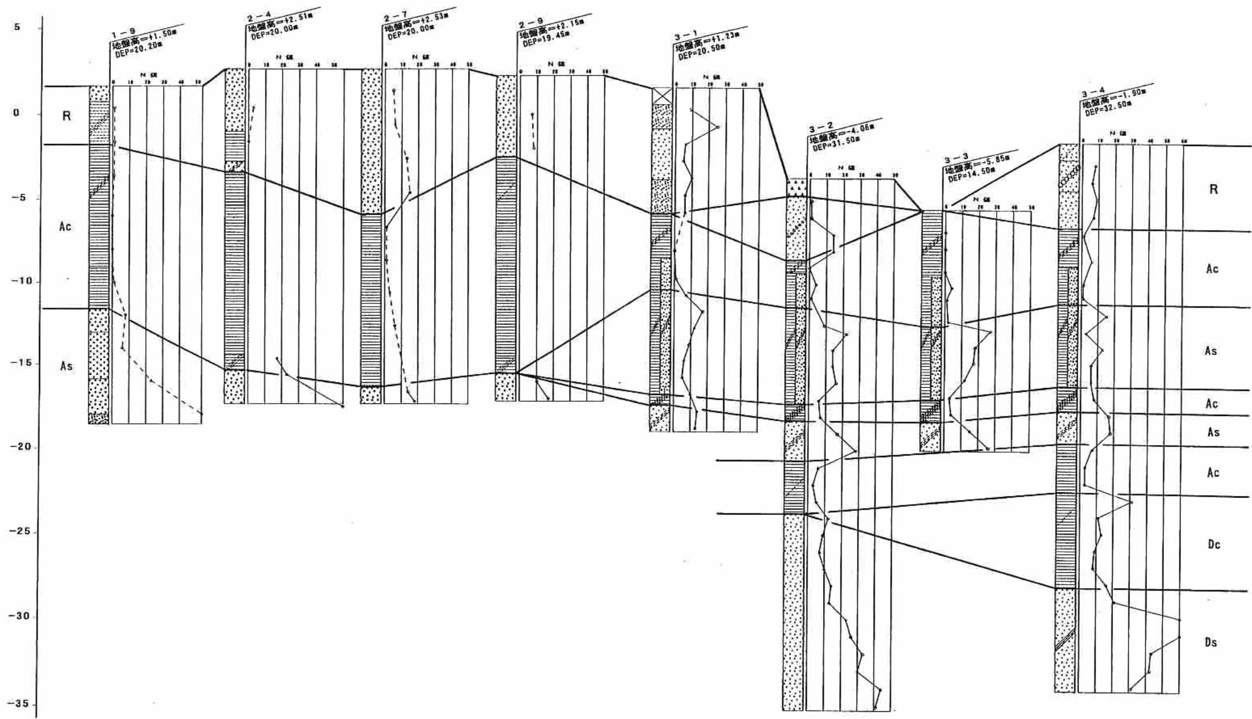
旗ヶ崎工業団地柱状図一覽図(既往-2)
