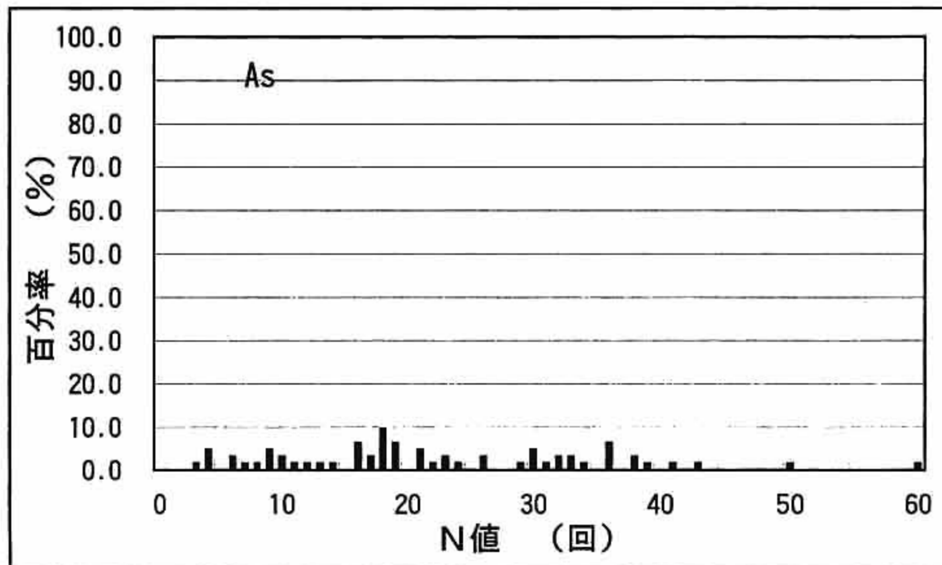
N値頻度分布図(崎津工業団地)
