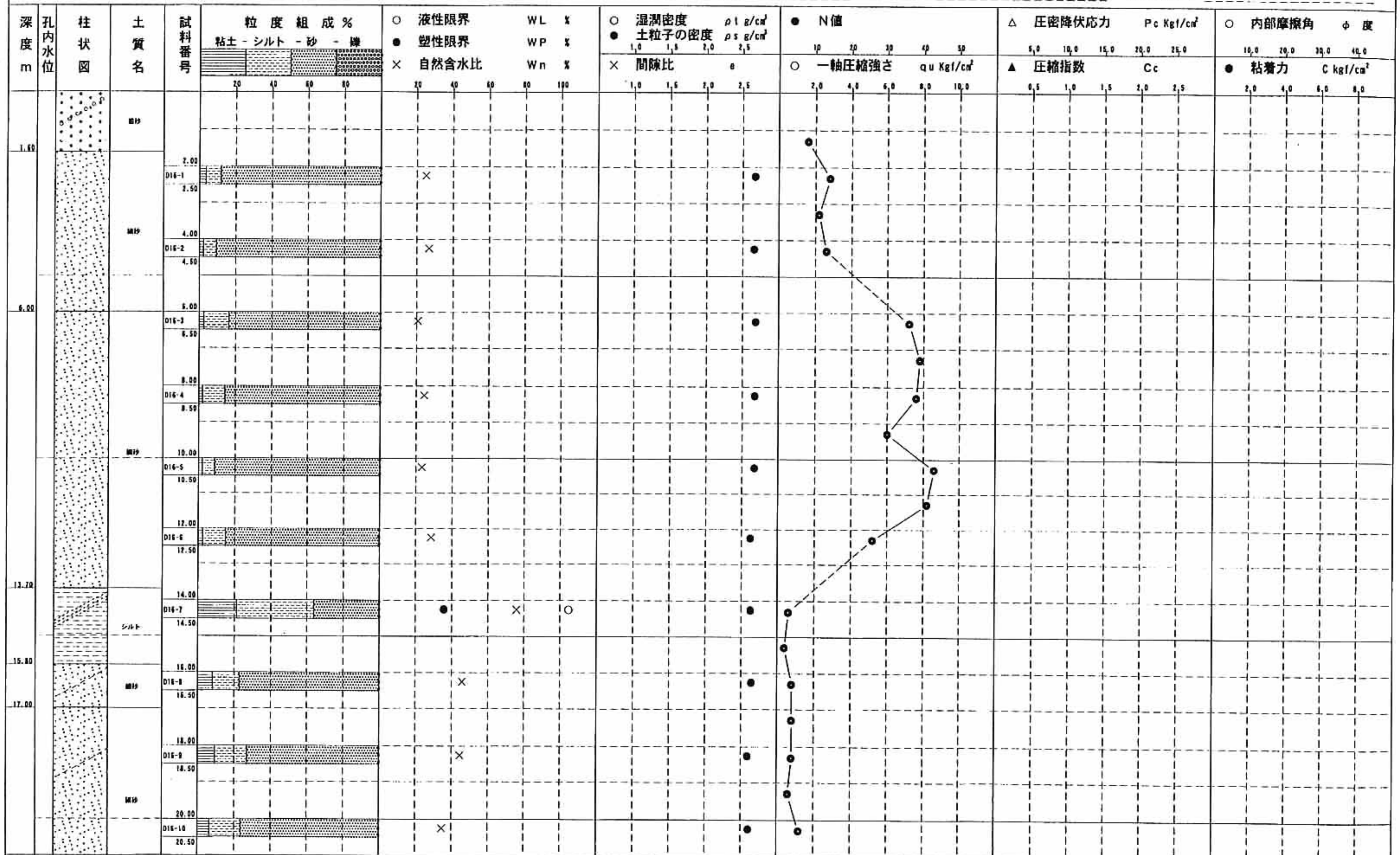
塑性図(崎津工業団地, B-12-16)
