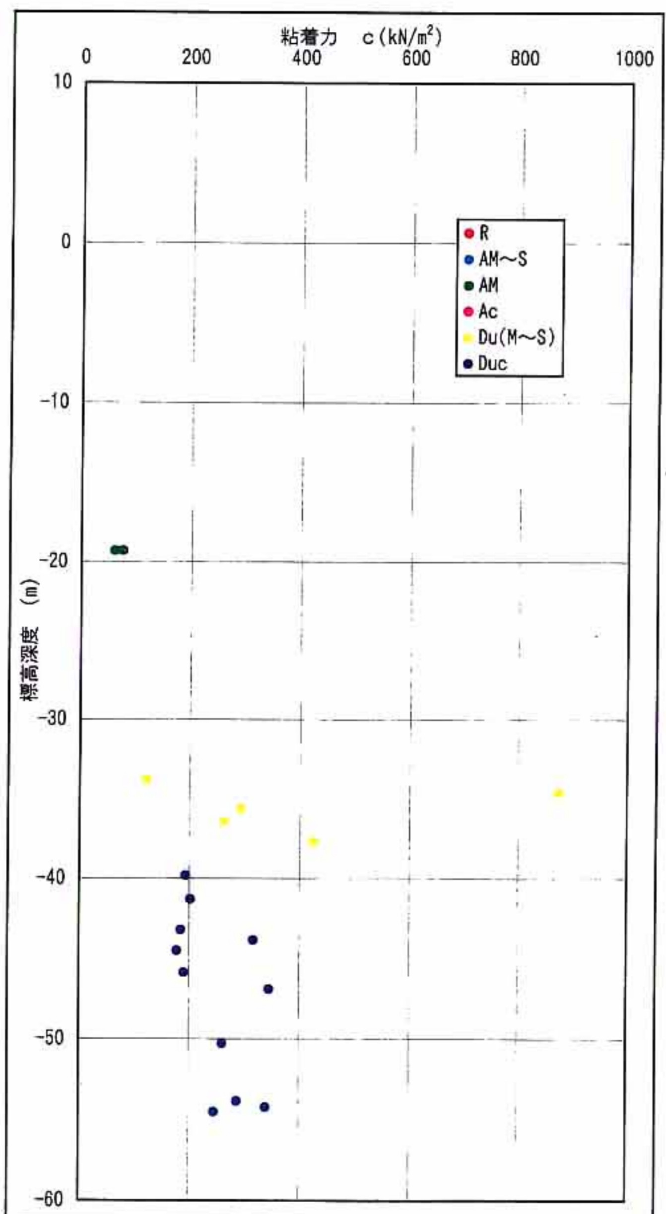
一軸圧縮強さ・粘着力・圧密降伏応力標高分布図(竹内工業団地)
