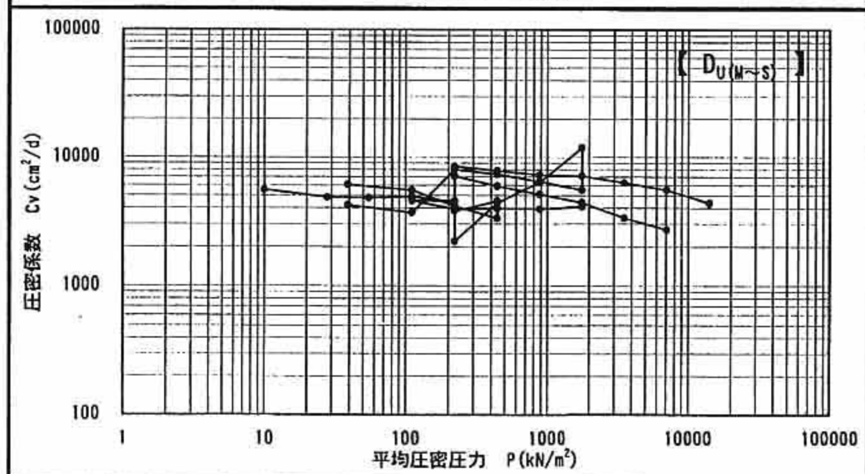
繰返し圧密試験結果図(竹内工業団地)
