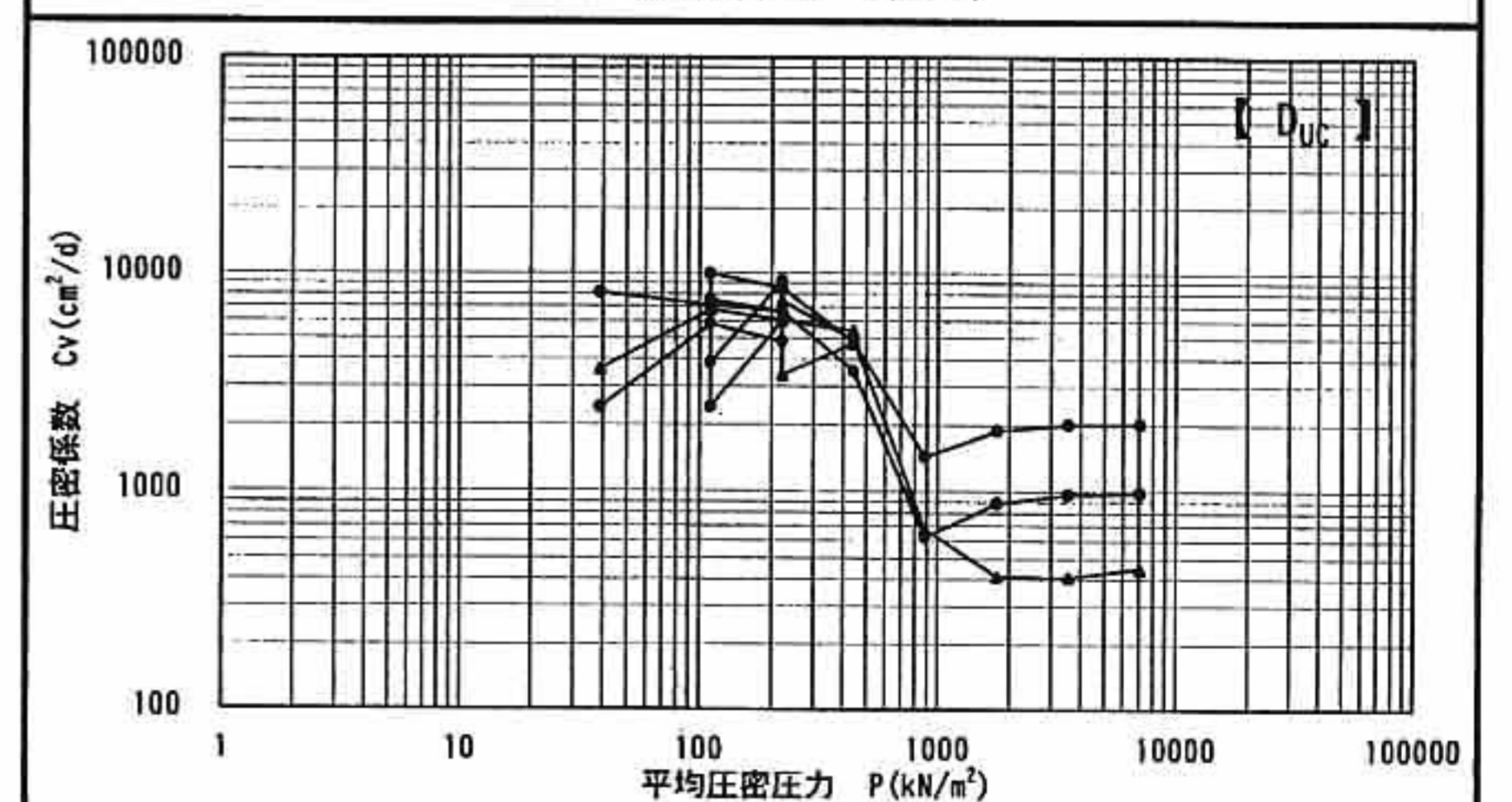
繰返し圧密試験結果図(竹内工業団地)
