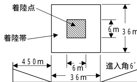
中型機(UH-1)の場合
