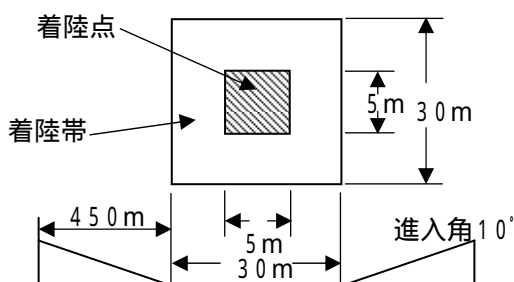
小型機(OH 6)の場合
