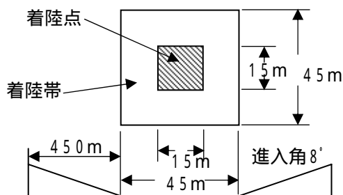
大型機(CH-47)の場合
