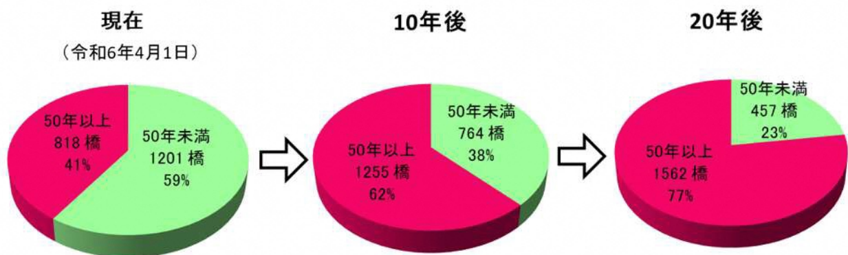
図 3.2 架設後の経過年数別橋梁数
