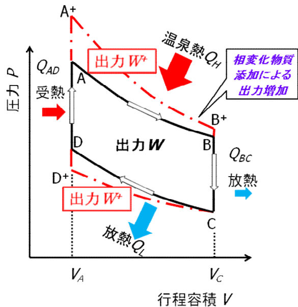
図 温泉熱駆動エンジンの出力
