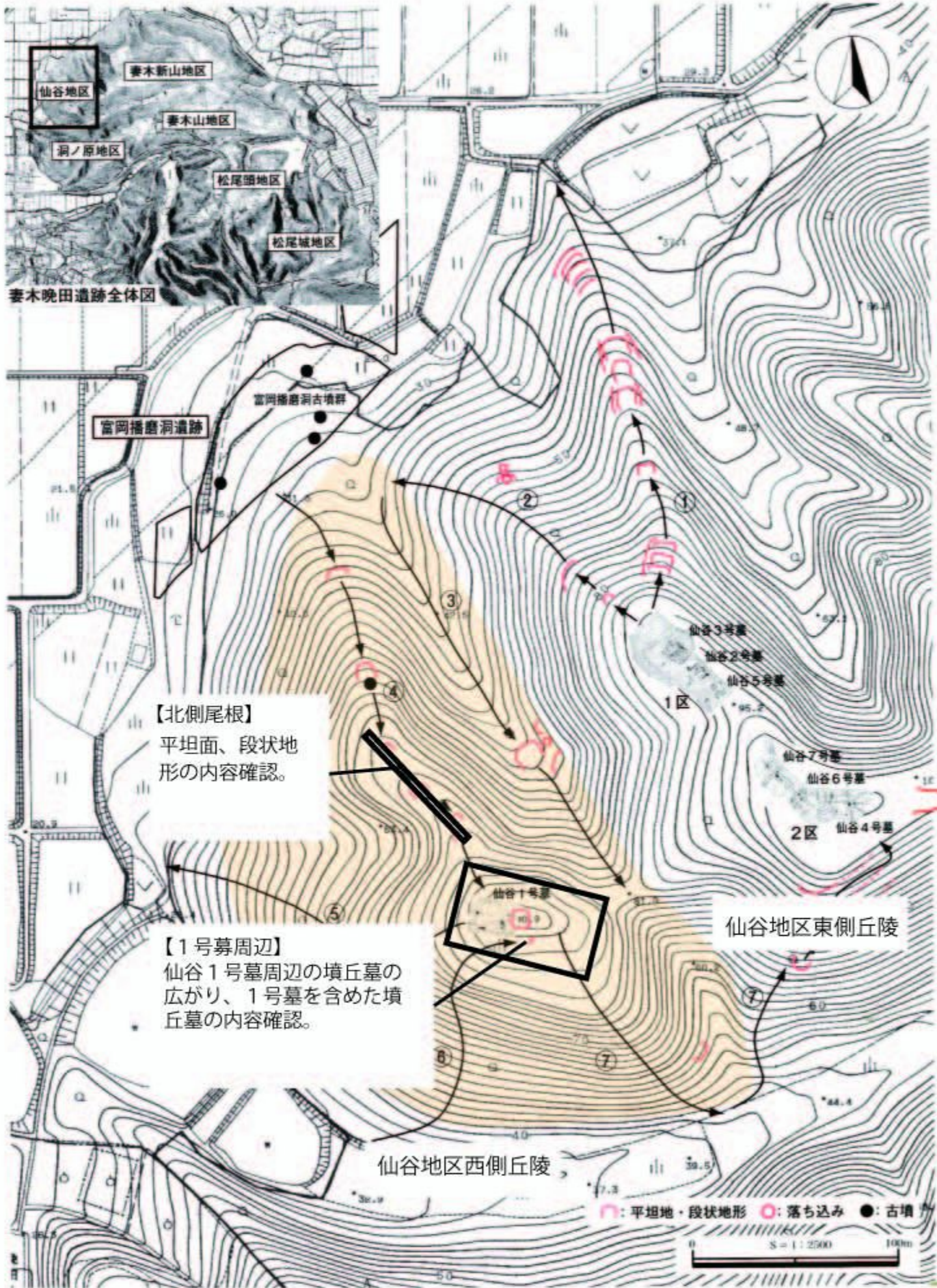
図1 仙谷地区西側丘陵調査計画図
