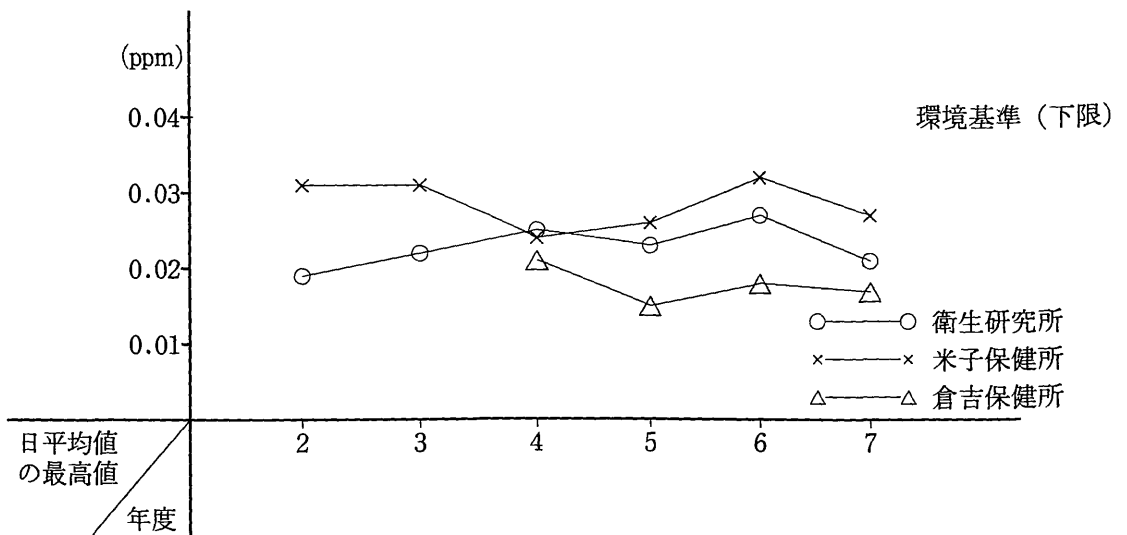
図5-1 二酸化窒素濃度経年変化（一般環境大気測定局）
