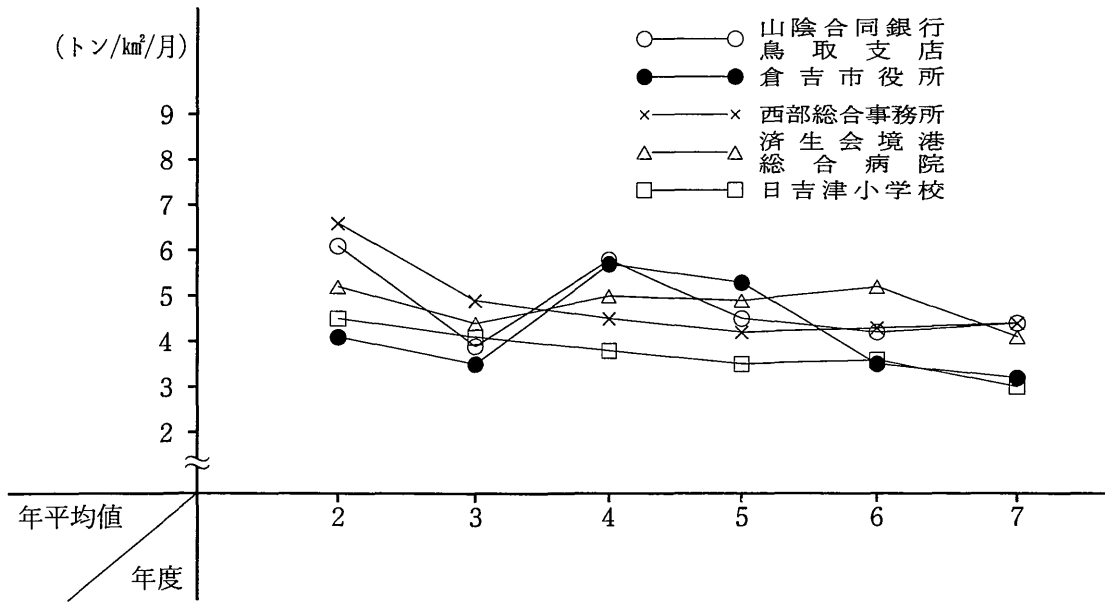
図8 降下ばいじん量の経年変化
