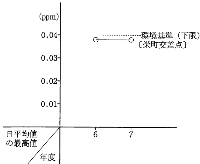
図5-2 二酸化窒素濃度経年変化（自動車排出ガス測定局）
