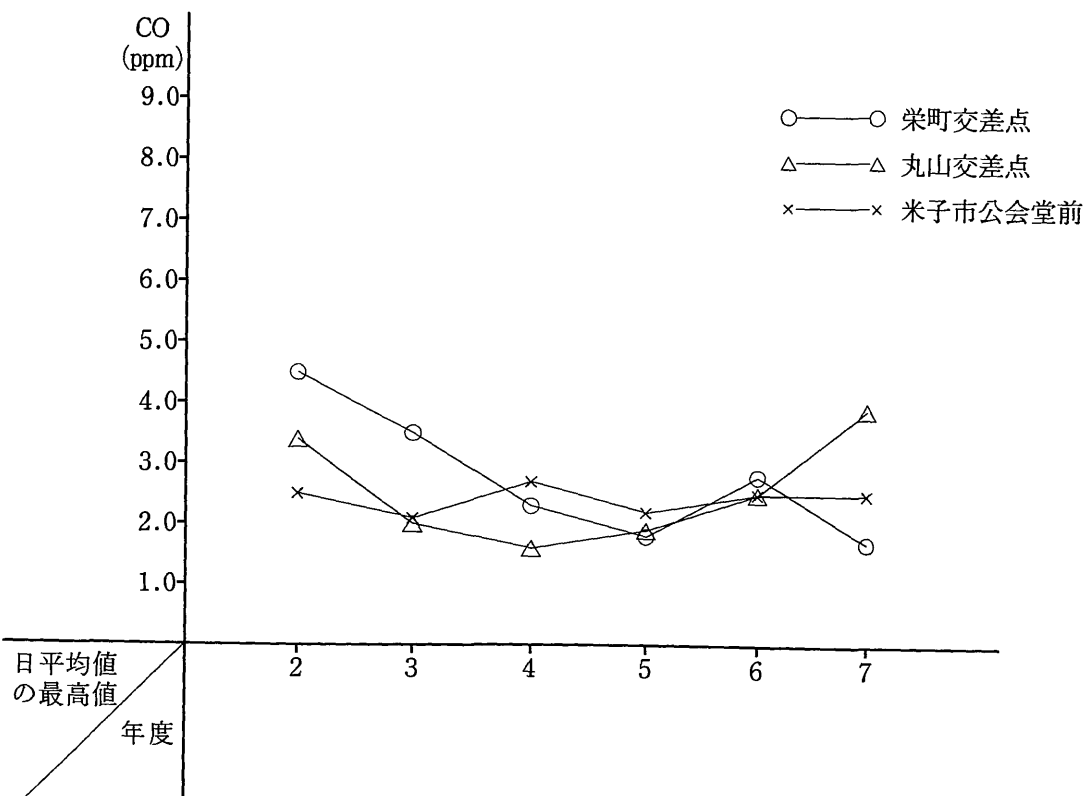
図3 一酸化炭素濃度経年変化（自動車排出ガス測定局）
