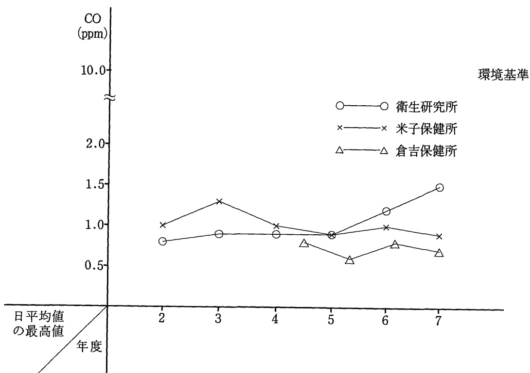
図2 一酸化炭素濃度経年変化（一般環境大気測定局）
