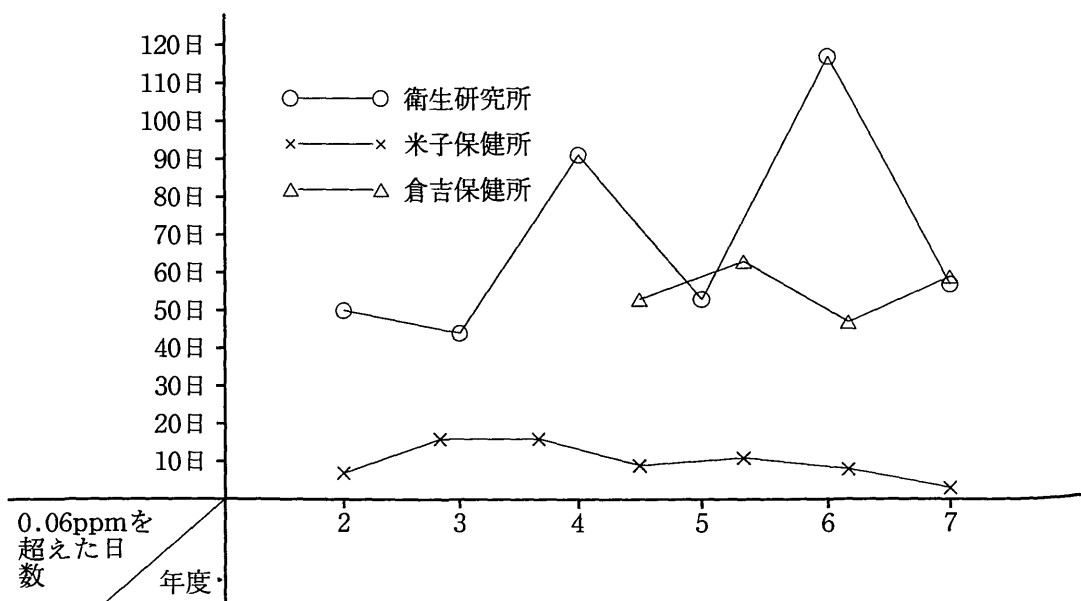
図6 光化学オキシダント環境基準を超えた日数の経年変化
