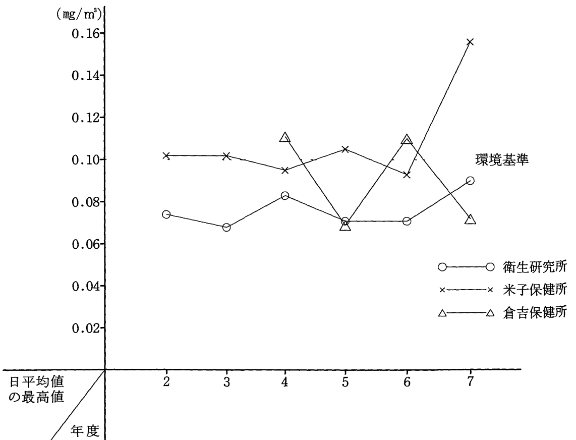
図4 浮遊粒子状物質濃度経年変化
