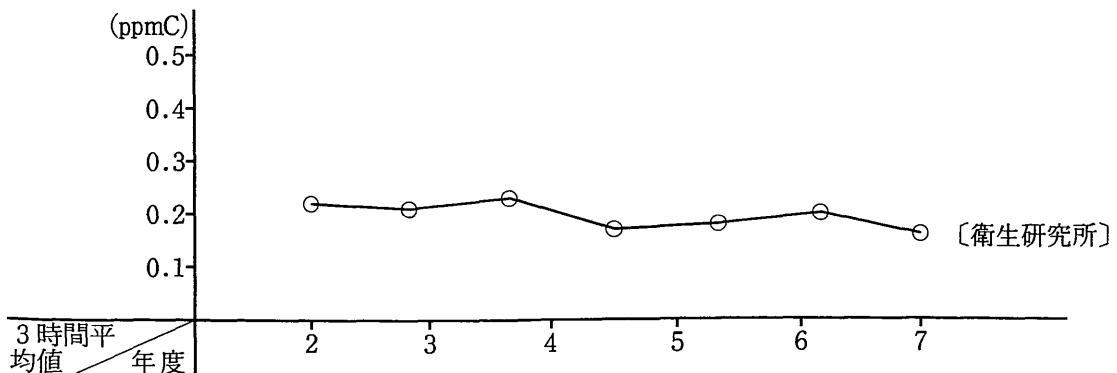
図7 非メタン炭化水素濃度経年変化
