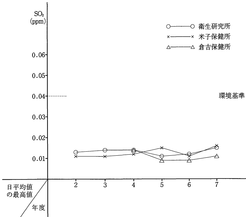
図1 二酸化いおう濃度の経年変化
