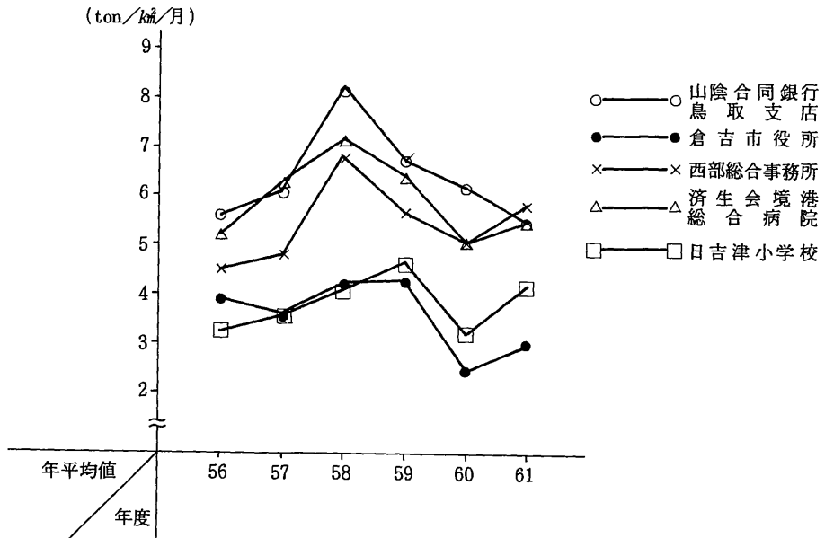
図8 降下ばいじん量の経年変化
