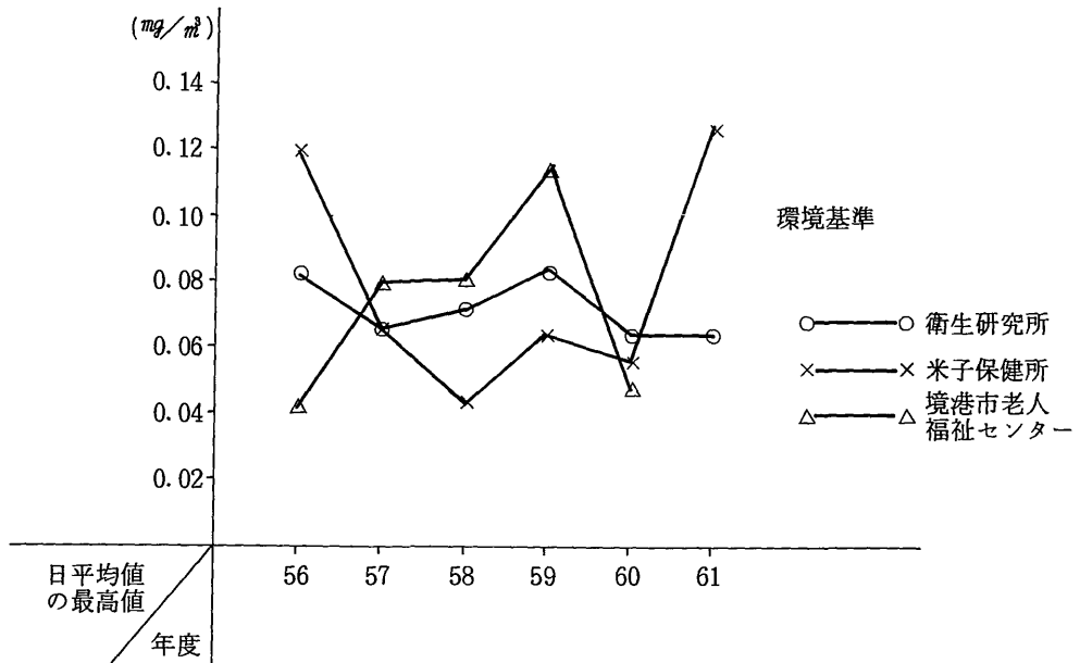
図5 浮遊粒子状物質濃度経年変化
