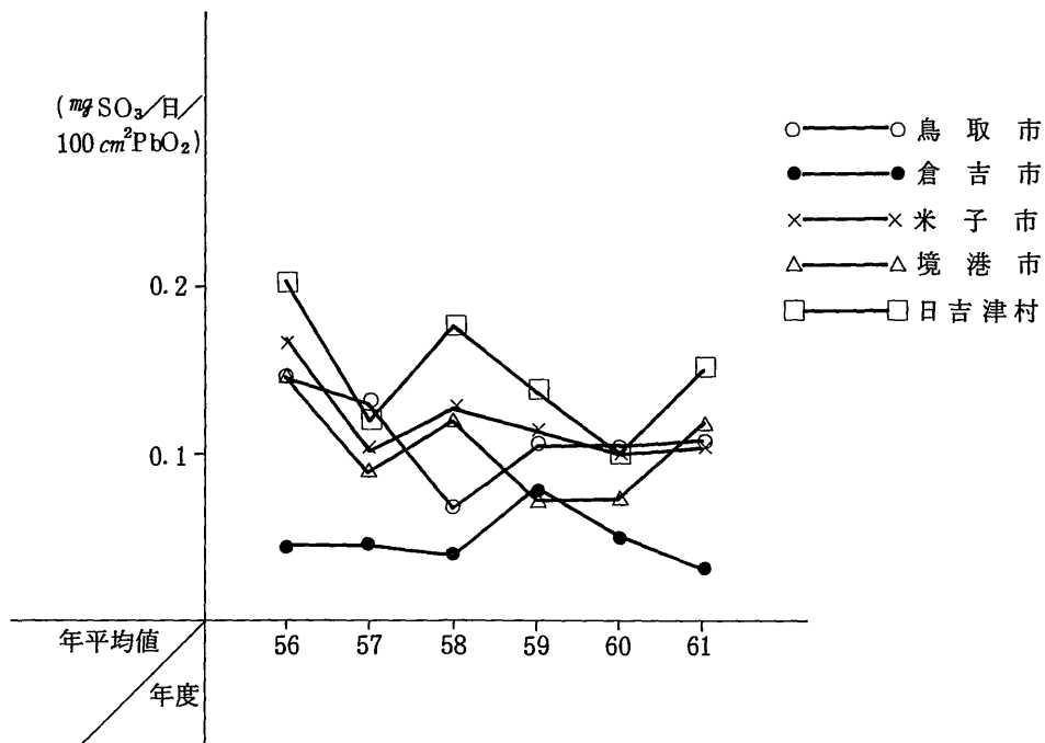
図2 二酸化鉛法による硫黄酸化物濃度経年変化
