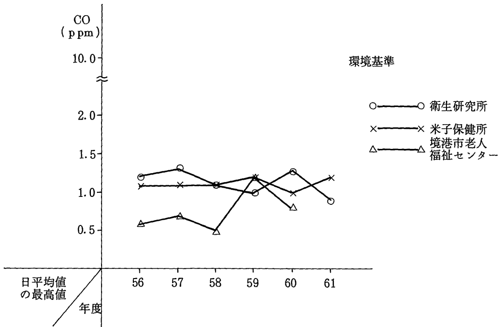
図4 一酸化炭素濃度経年変化(自動車排出ガス測定局)
