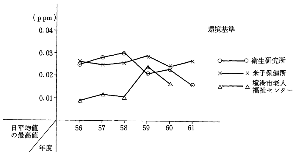
図6 二酸化窒素濃度経年変化
