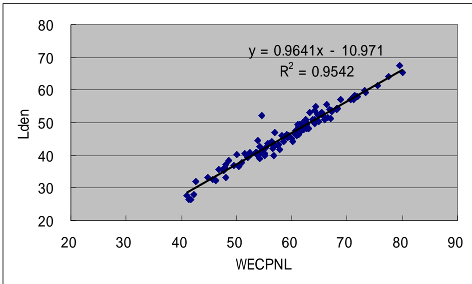
図3 美保飛行場周辺におけるWECPNLとLdenの関係 (N=112)
