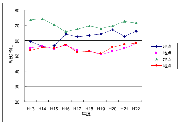
図2 各地点別のWECPNLの経年変化図
