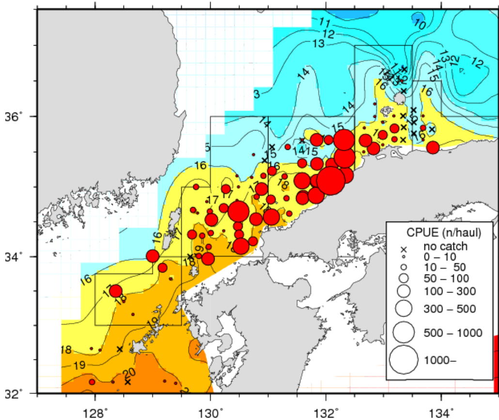
図 1 2012 年のトロール網調査結果 円の大きさはマアジの採集量の多さを表し、×は採集されなかった点を表す。実線の等温線は水深 50m の水温分布を表す。
