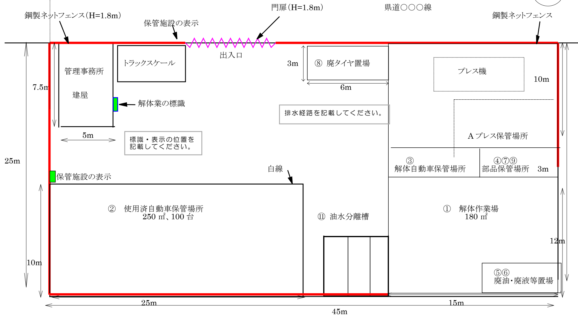
施設配置図 (S=1:200)
