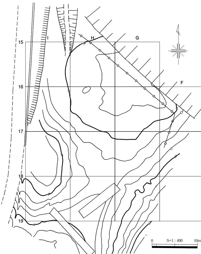
第5図 調査前地形測量図
