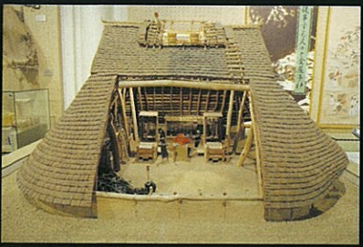
高殿模型 和鋼博物館(安来市)蔵 本床にある高殿で鉄が精錬された
