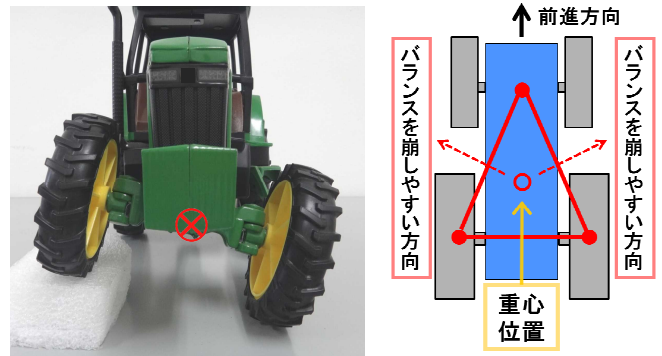
図2. トラクターの重心位置
