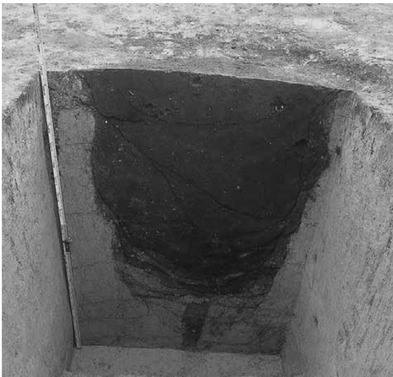
1 SK18土層断面(北西から)
