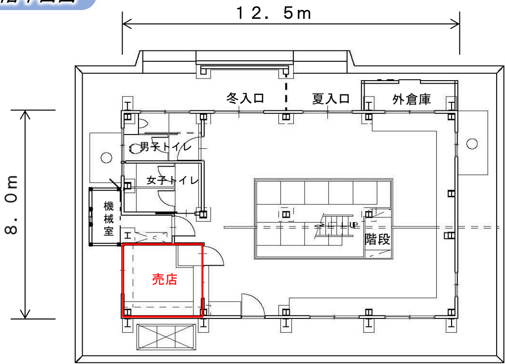
1 階平面図
