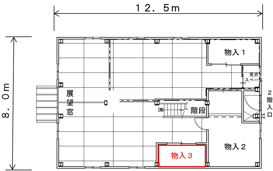
2 階平面図
