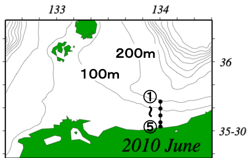
図1) 6月25日の水温の鉛直断面図
